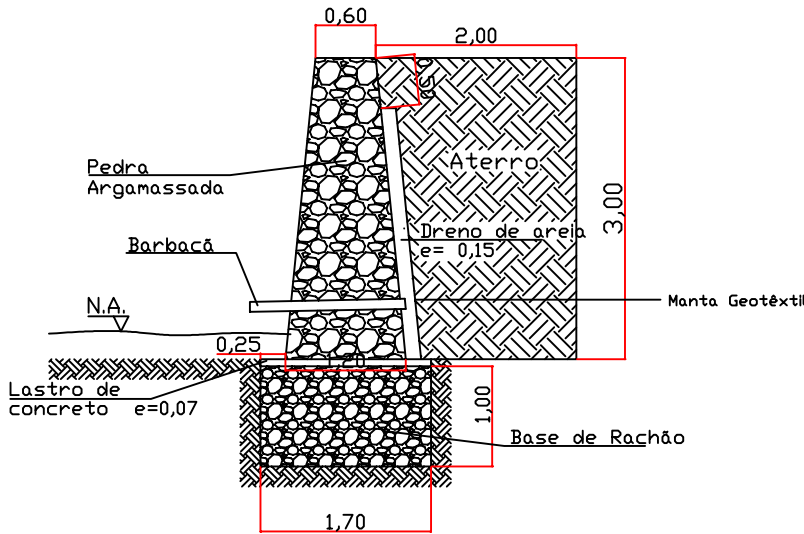
DETALHE CONSTRUTIVO
