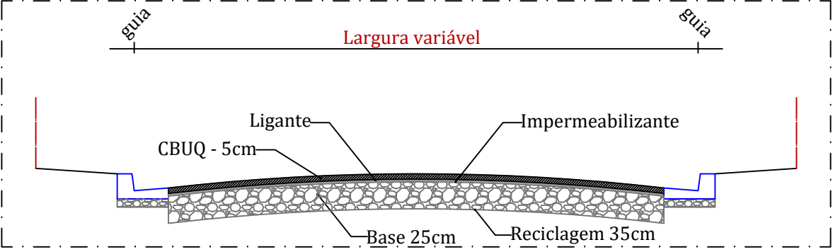
Perfil Pavimentação (Largura variável) sem escala
