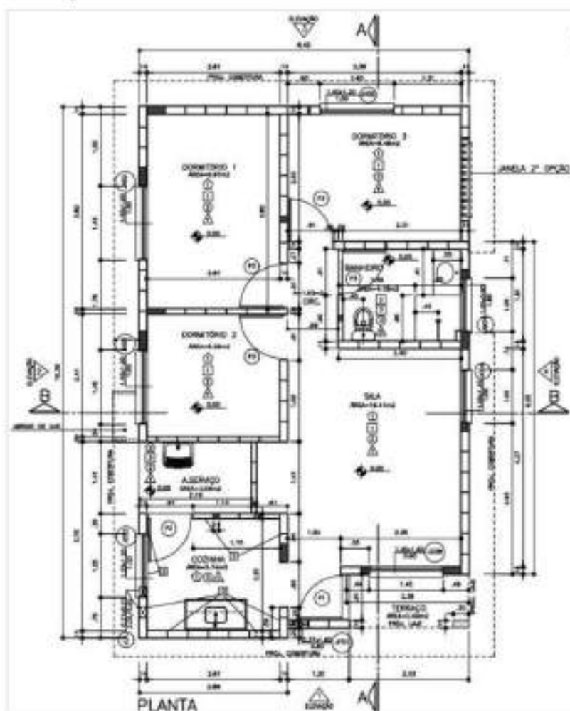
Figura 1 – Planta esquemática, tipologia T133B - 03, com opção de três dormitórios.
