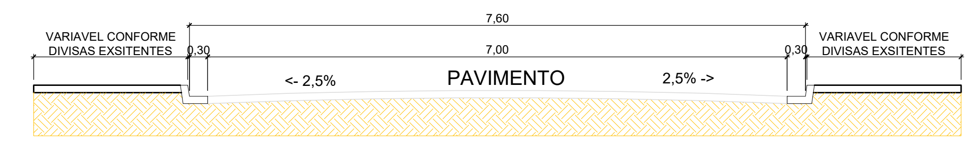
PERFIL DO PAVIMENTO
