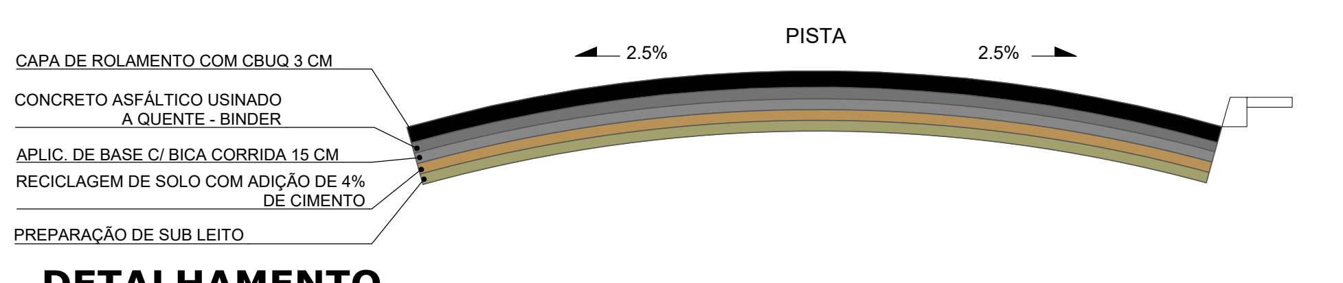
DETALHAMENTO
