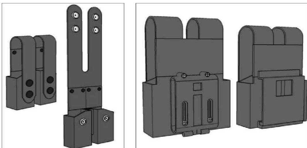
Figura 3: À esquerda, visualização em perspectiva do porta-carregadores em polímero de alta resistência com a tampa fechada e aberta. À direita, passadores de acoplamento ao cinturão em dobradiça ou travamento por ponto de encaixe.
