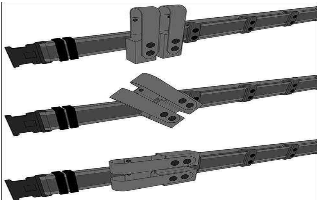
Figura 02: Posições de ajuste do porta carregadores (vertical, angular e horizontal).
