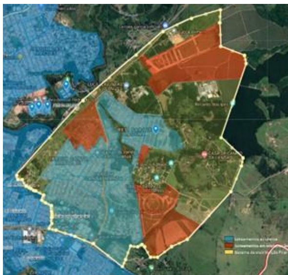
Fig. 08: Setorização do Sistema de distribuição Pirai.
