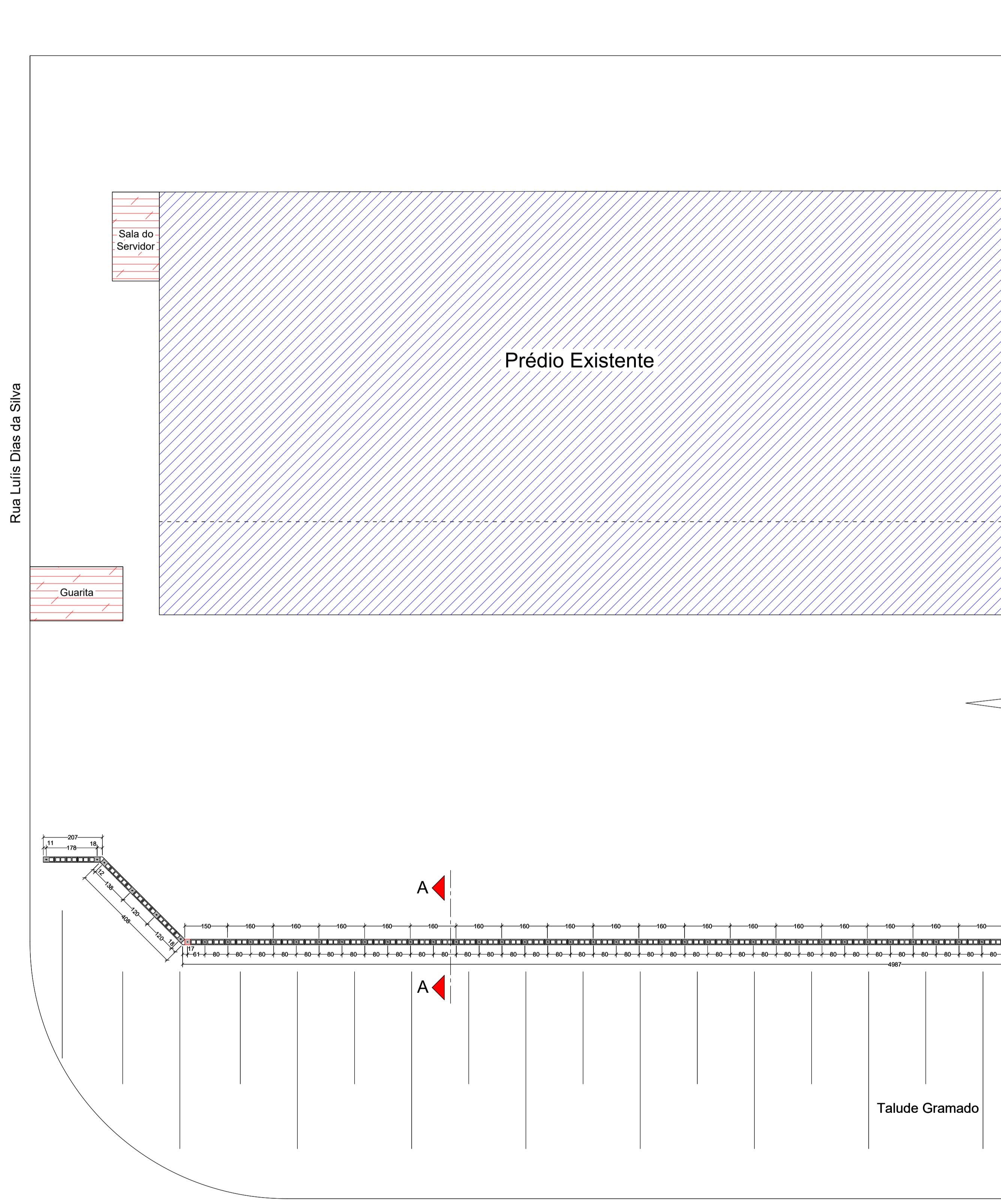
Planta de Forma de Distribuição das Fiadas - Muro Arrimo - Parte A Escala: 1/50 Dimensões em Centímetros
