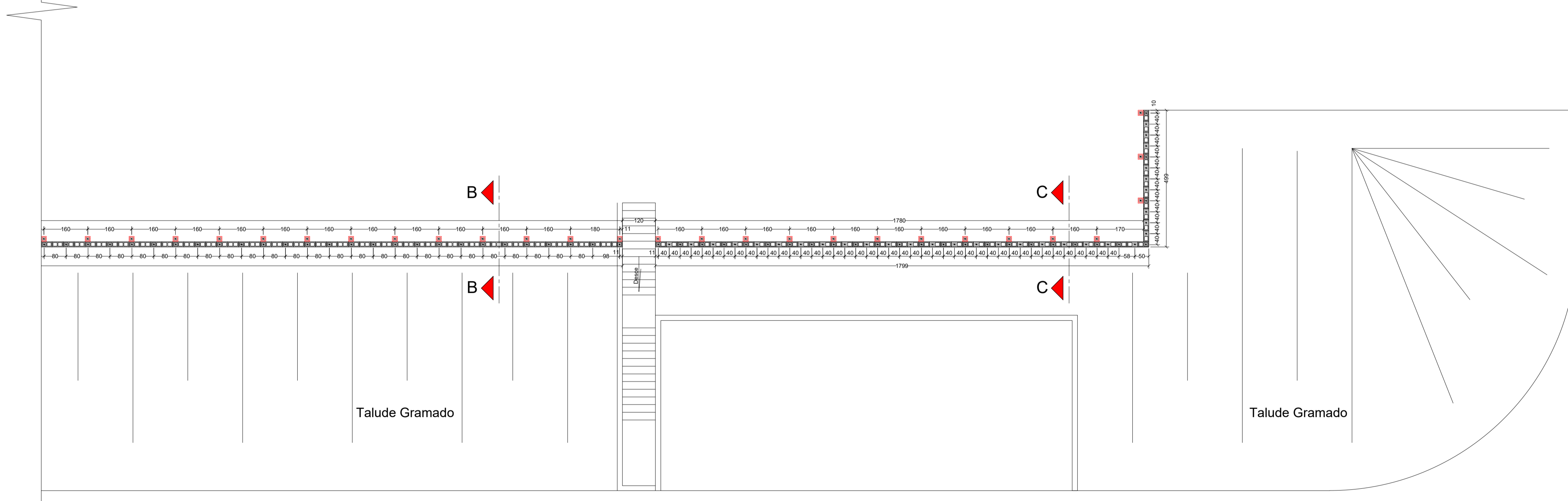
Planta de Forma de Distribuição das Fiadas - Muro Arrimo - Parte B Escala: 1/50 Dimensões em Centímetros
