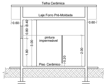
Corte BB esc: 1/50
