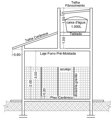
Corte AA esc: 1/50
