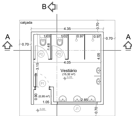
Planta Baixa esc: 1/100
