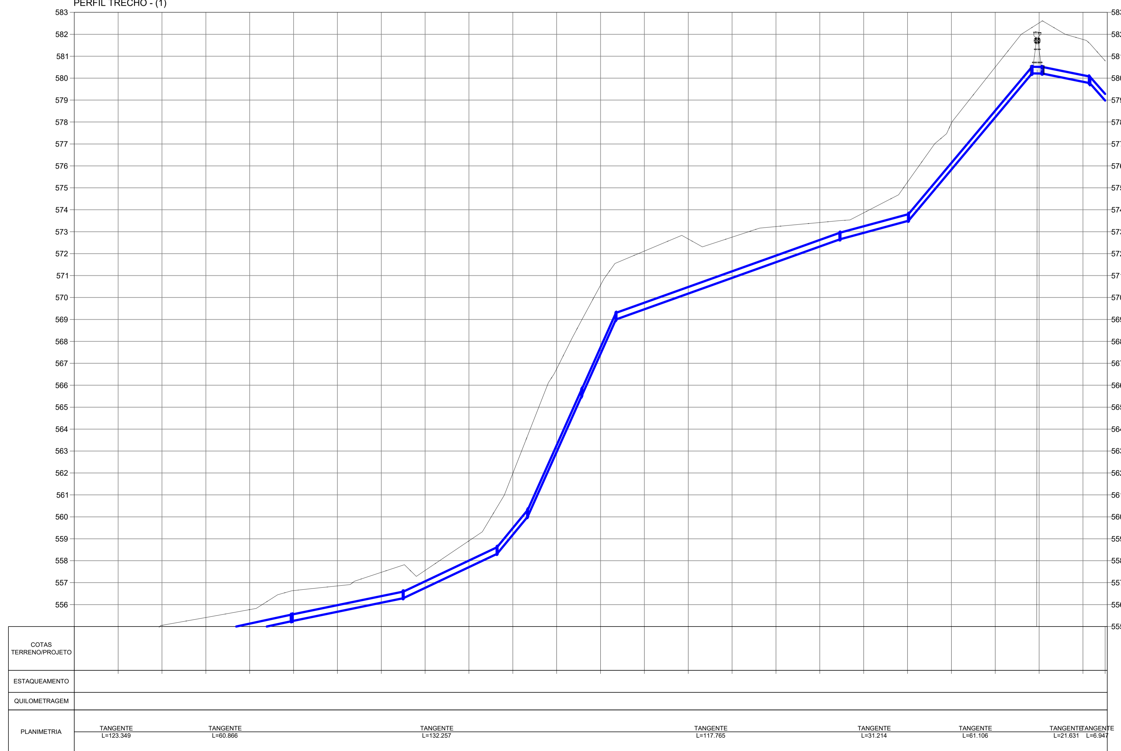
PERFIL TRECHO - (1)
