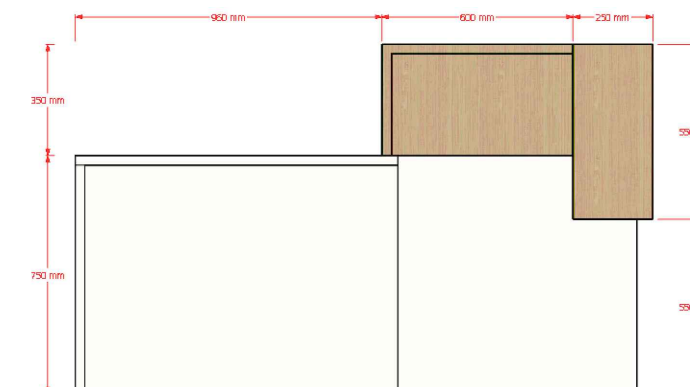
VISTA 04 SEM ESCALA
