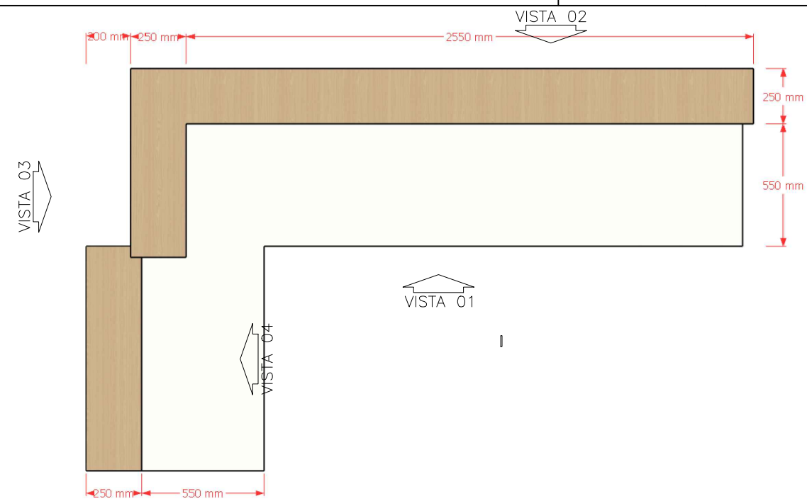
PLANTA BAIXA - BALCÃO SEM ESCALA
