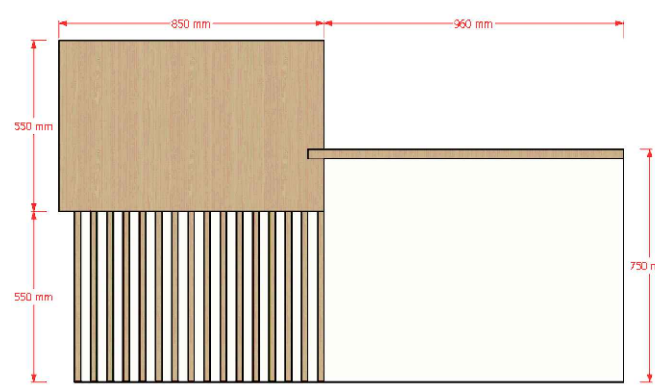
VISTA 03 SEM ESCALA
