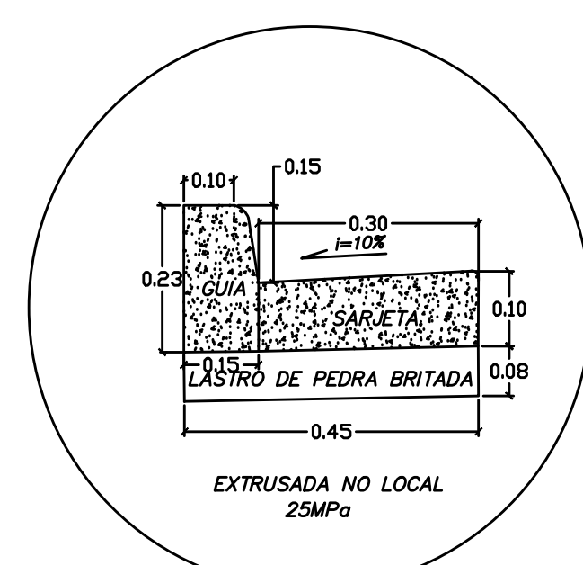
DETALHE GUIAS E SARJETAS SEM ESCALA
