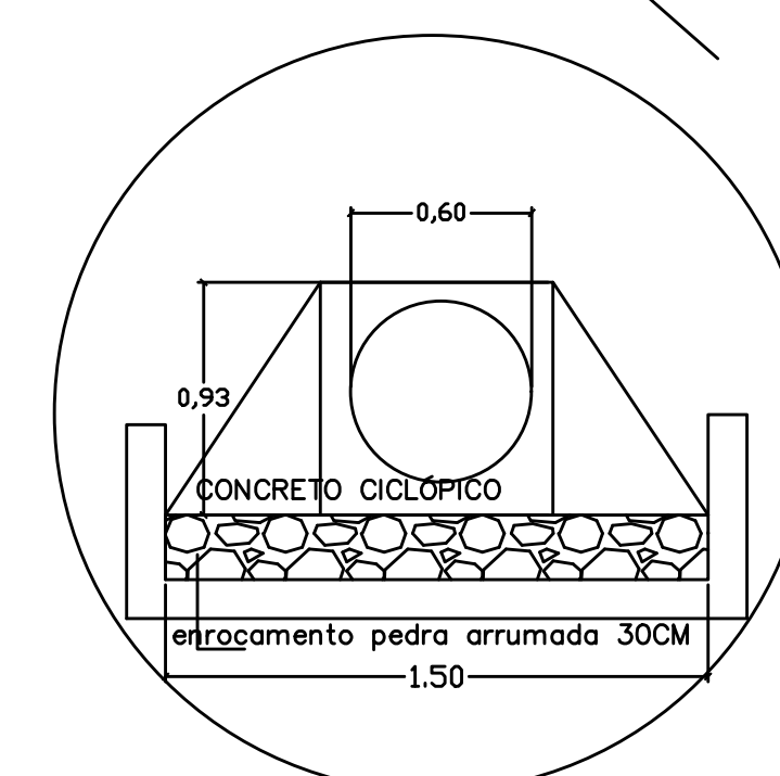
DETALHE MURO DE ALA E CAIXA DE DETA
