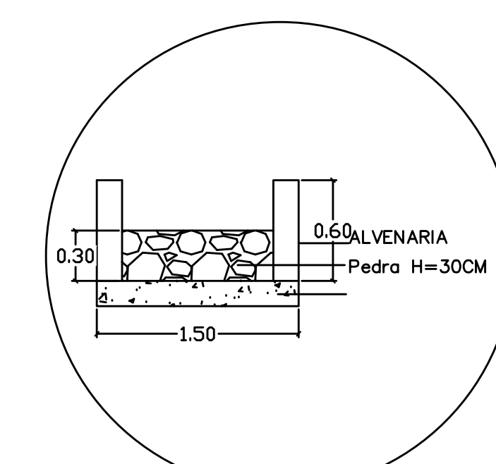
DETALHE MURO DE ALA E CAIXA DE FETRA
