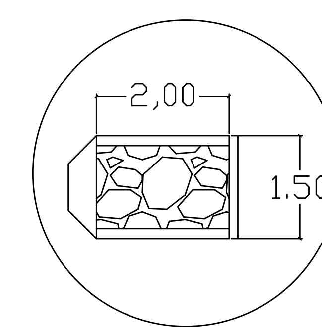
DETALHE MURO DE ALA E CAIXA DE PEDRA
