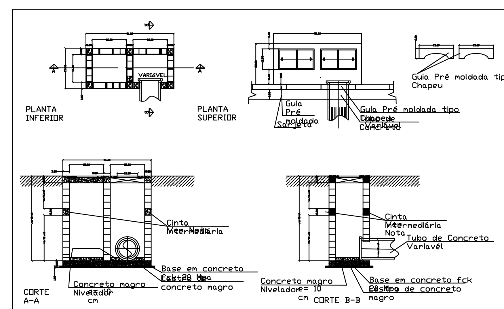
DETALHE DA BOCA DE LOBO DUPLA
