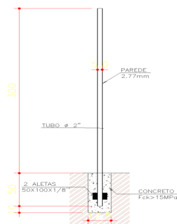
DETALHE "B" FIXAÇÃO NO SOLO SEM ESCALA
