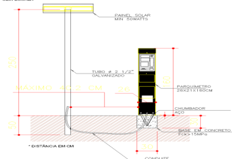
DETALHE “F” VISTA FRONTAL DO PARQUÍMETRO SEM ESCALA
