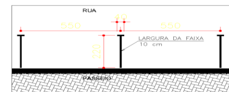
DETALHE "C" SINALIZAÇÃO HORIZONTAL SEM ESCALA - MEDIDAS EM CM
