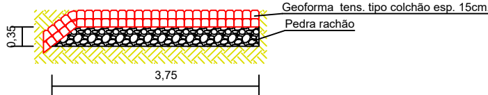
DETALHE DA MELHORIA DE SUB-LEITO / SUPORTE Escala:- Sem escala.
