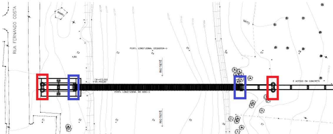
Imagem 02: Implantação Passarela Pênsil com destaque em vermelho dos tubulões existentes nos quais deverão ser realizadas as provas de carga horizontal e com destaque em azul os tubulões existentes nos quais deverão ser realizadas as provas de carga vertical.
