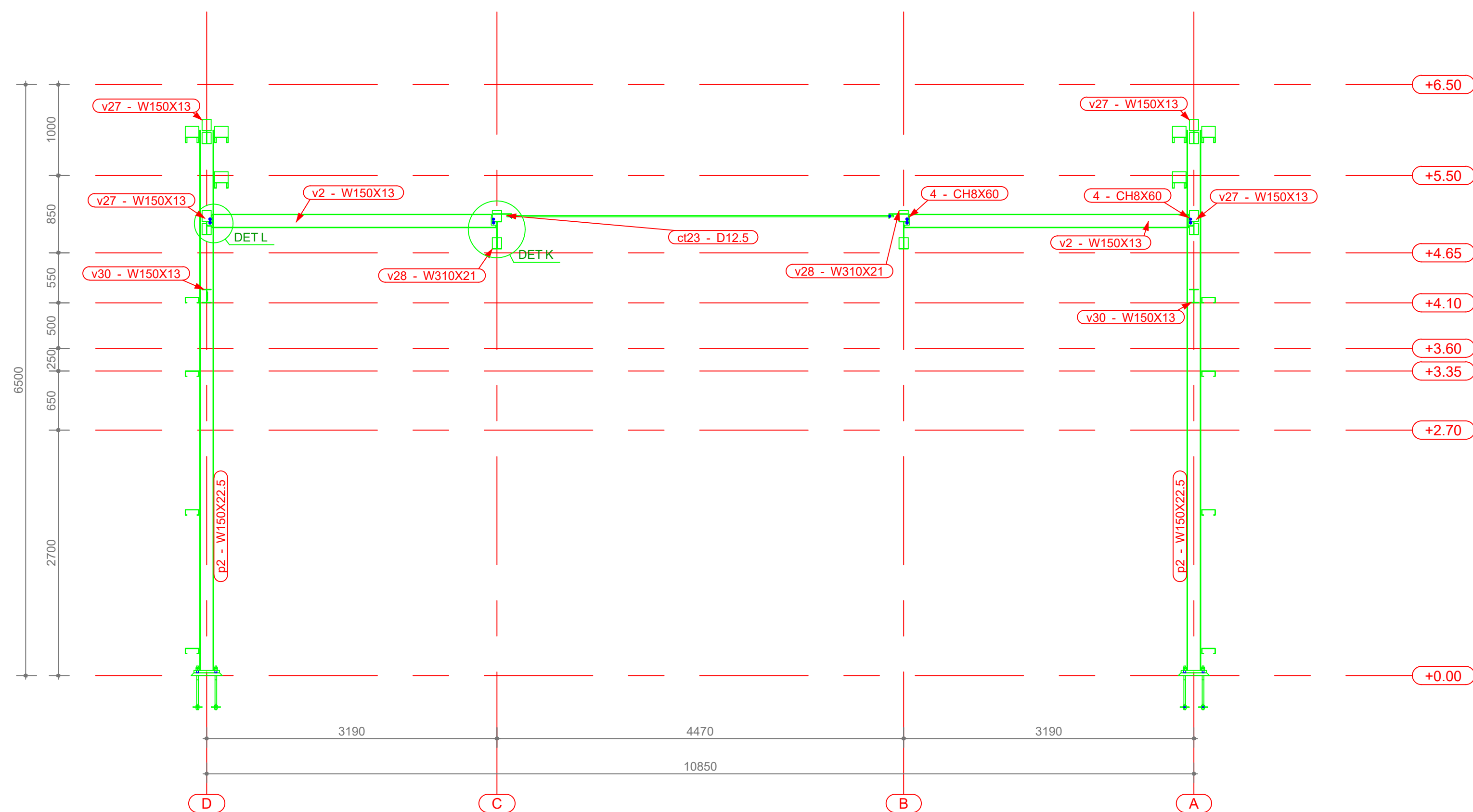
EIXO 2 Escala: 1:40
