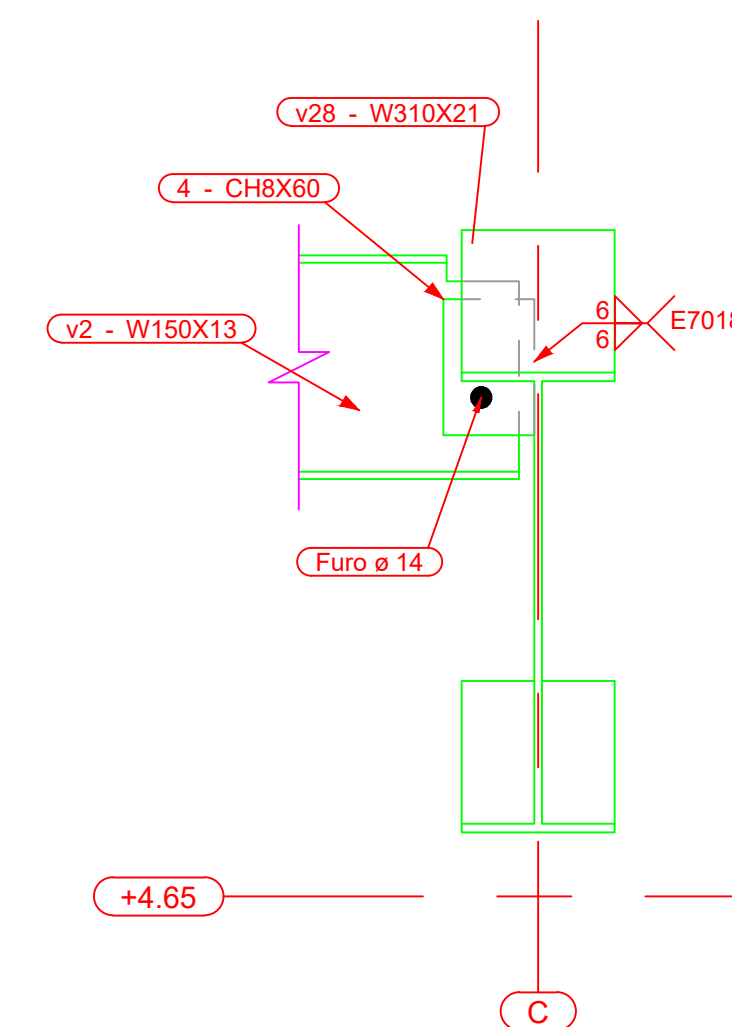
DETALHE K Esc: 1:5
