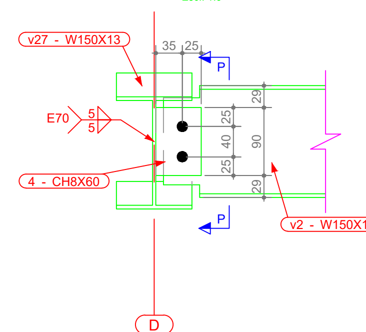
DETALHE L Esc: 1:5
