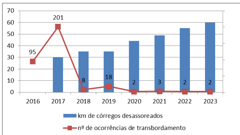
Gráfico 1 - O aumento da extensão (km) do contrato de desassoreamento coincide com uma sensível redução nas ocorrências de transbordamento dos córregos.
