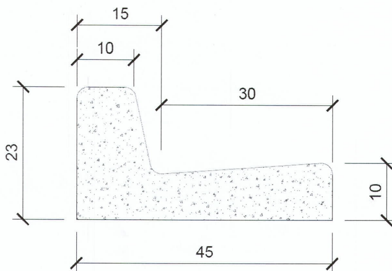
Figura 1 - Dimensões do conjunto guia e sarjeta
