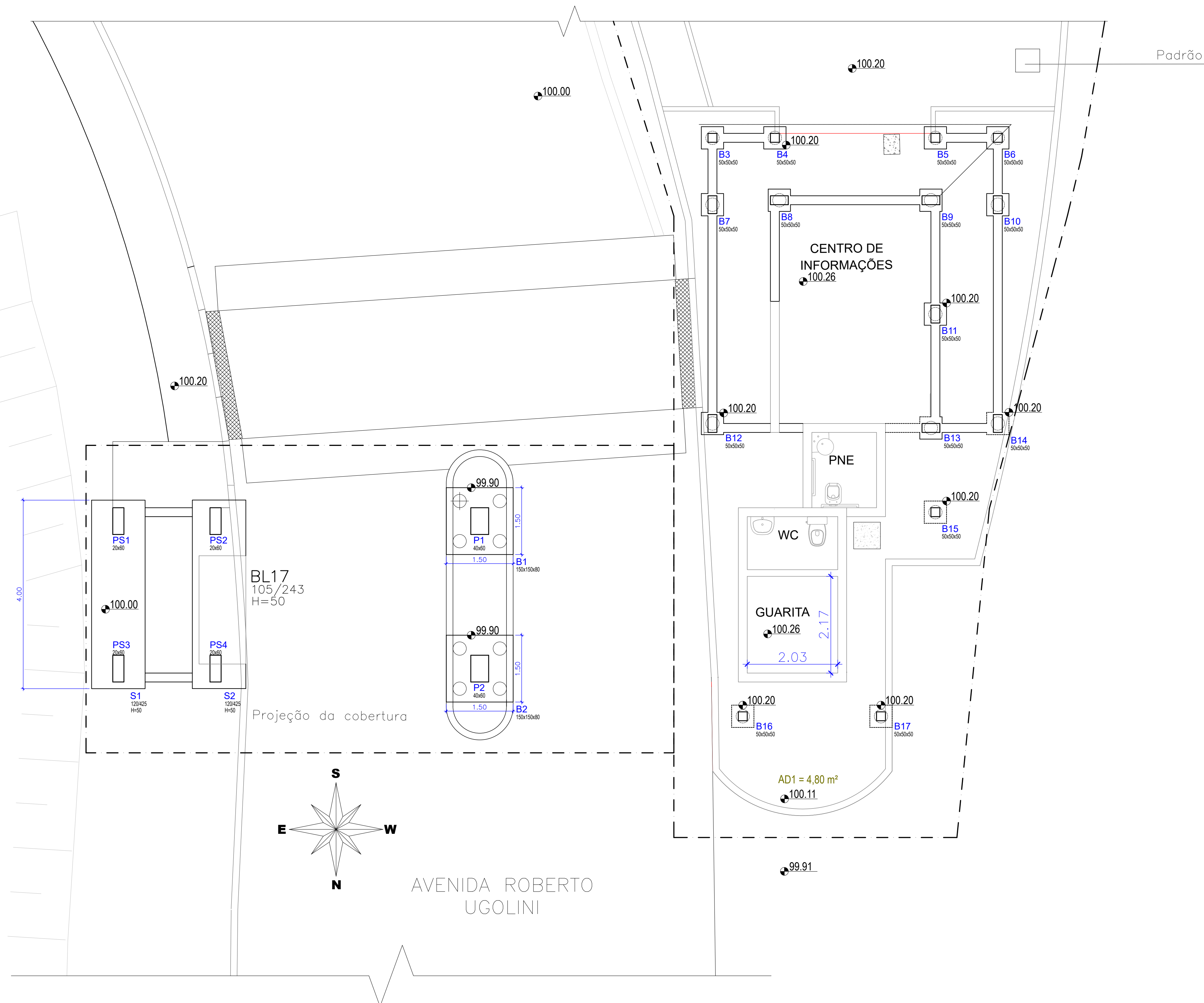
PLANTA DE FUNDAÇÃO: FÔRMA ESCALA: 1:50
