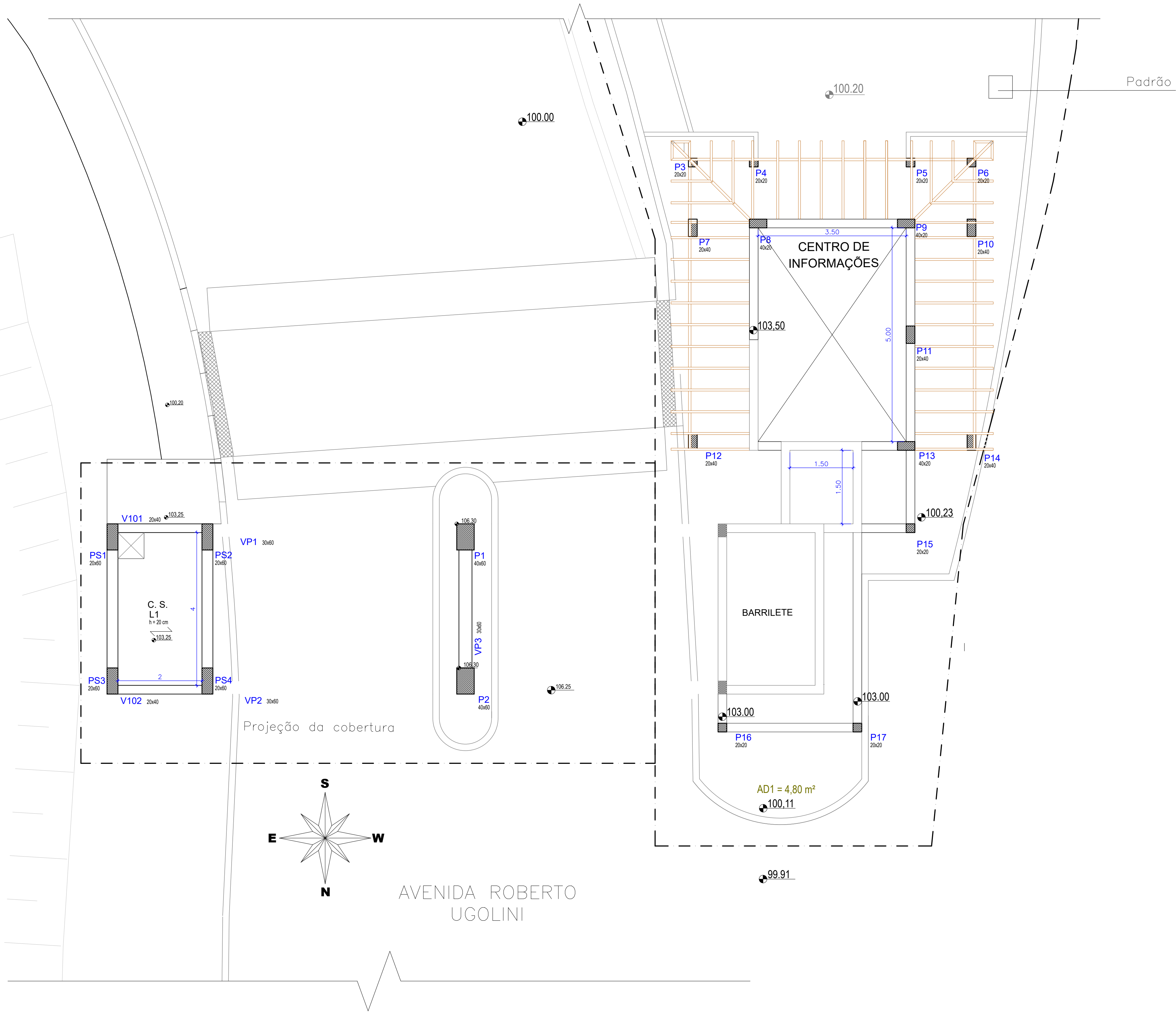
PLANTA DE ESTRUTURA: PAVIMENTO SUPERIOR ESCALA: 1:50
