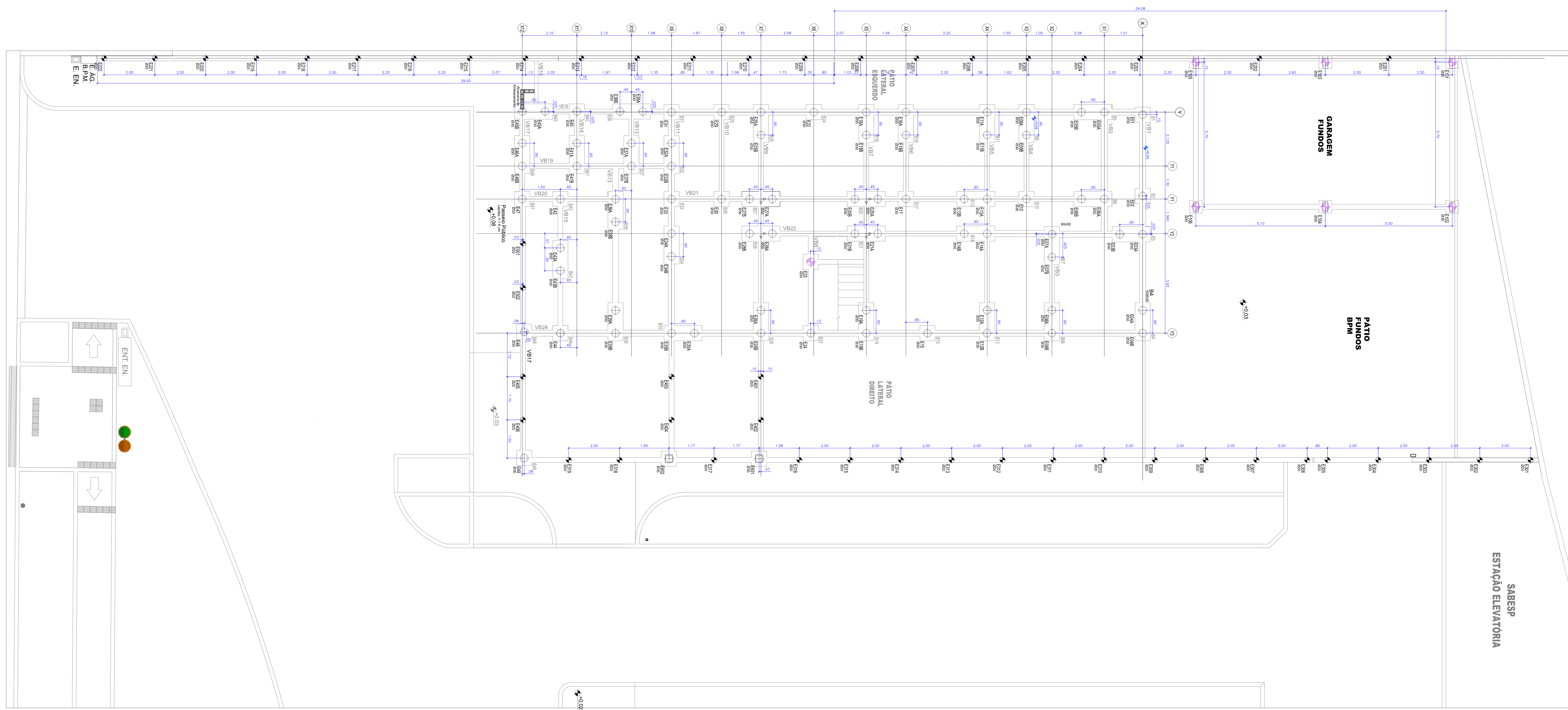
FUNDAÇÃO: LOCAÇÃO DAS ESTACAS ESC. 1/50
