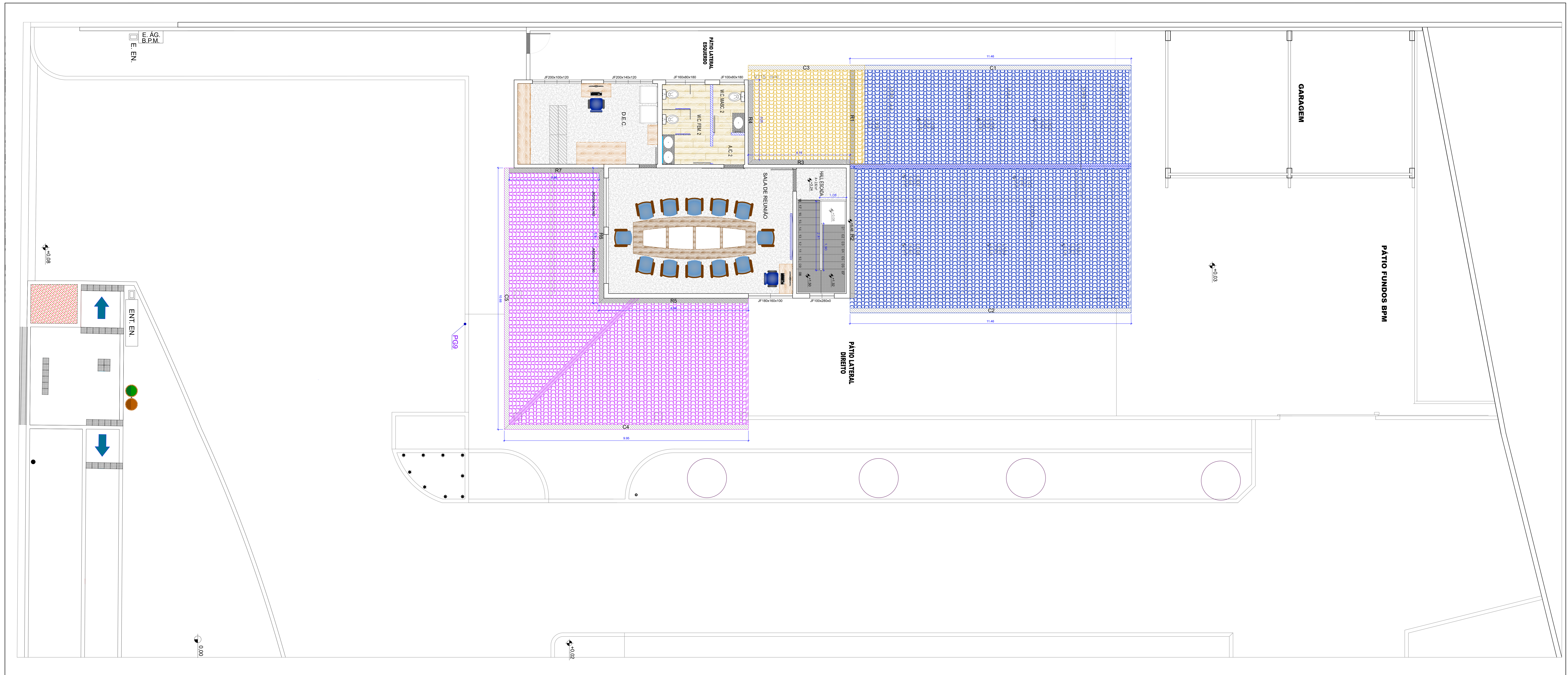
ARQUITETURA: PRIMEIRO PAVIMENTO - PLANTA DE LAYOUT ESCALA: 1-50
