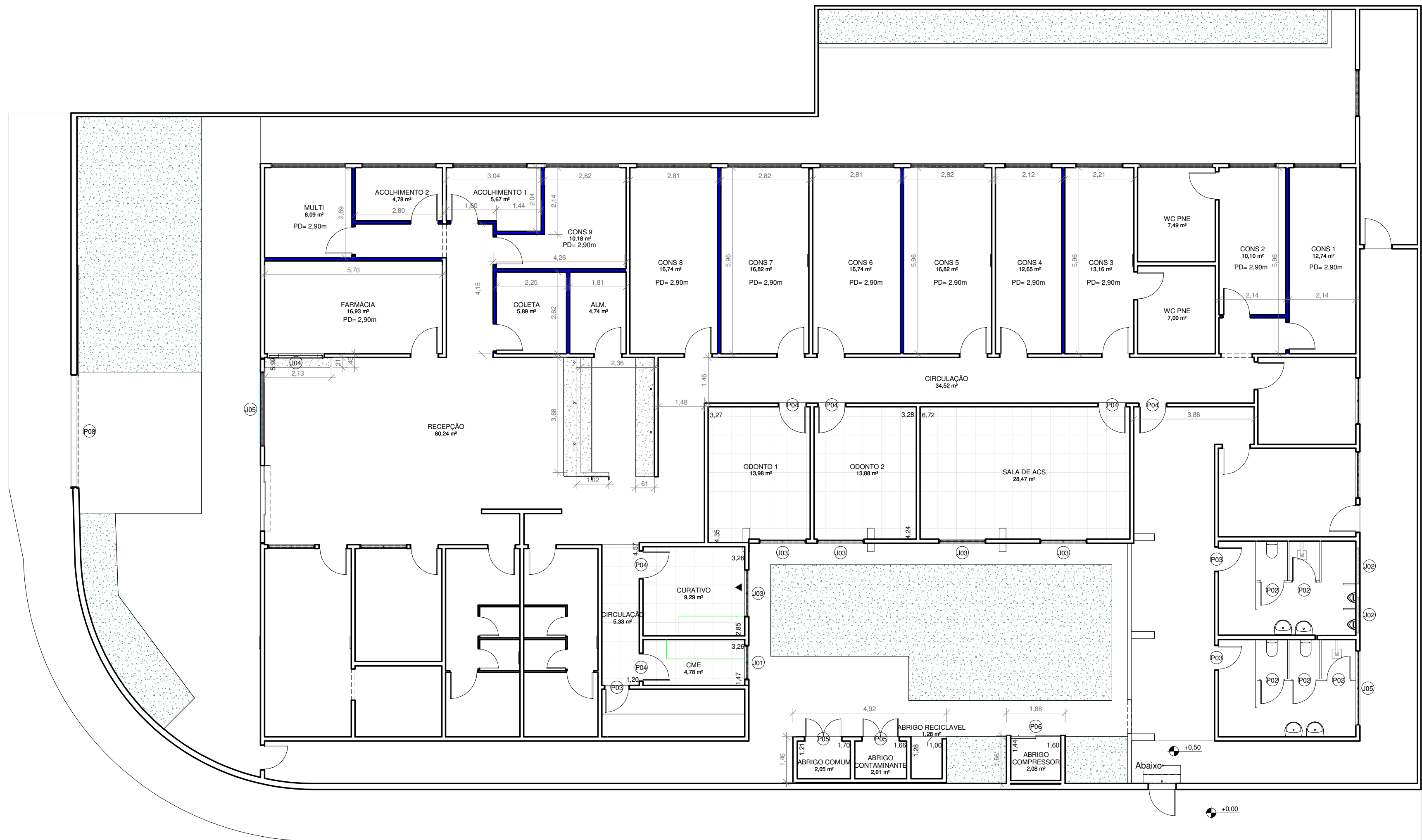
1 TÉRREO - LAYOUT ESCALA 1 : 100 LEGENDA ■ DRYWALL
