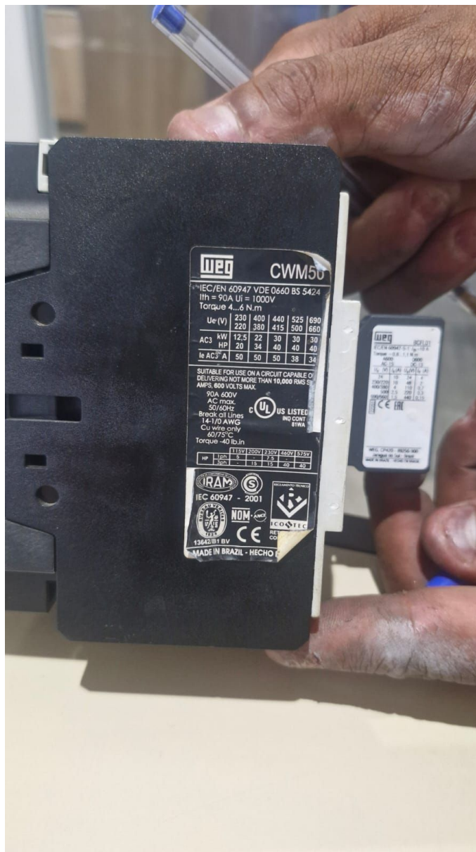
Imagem 01 – Contator WEG CWM50 e bloco auxiliar instalados no equipamento existente, utilizados como referência para compatibilidade técnica.
