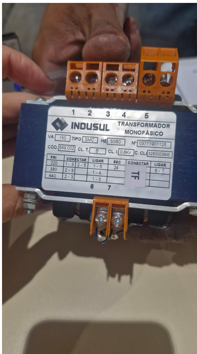
Imagem 02 – Transformador monofásico INDUSUL, 150 VA, com primário 220/380/440 V e secundário 24 V, instalado no equipamento existente, utilizado como referência técnica.
