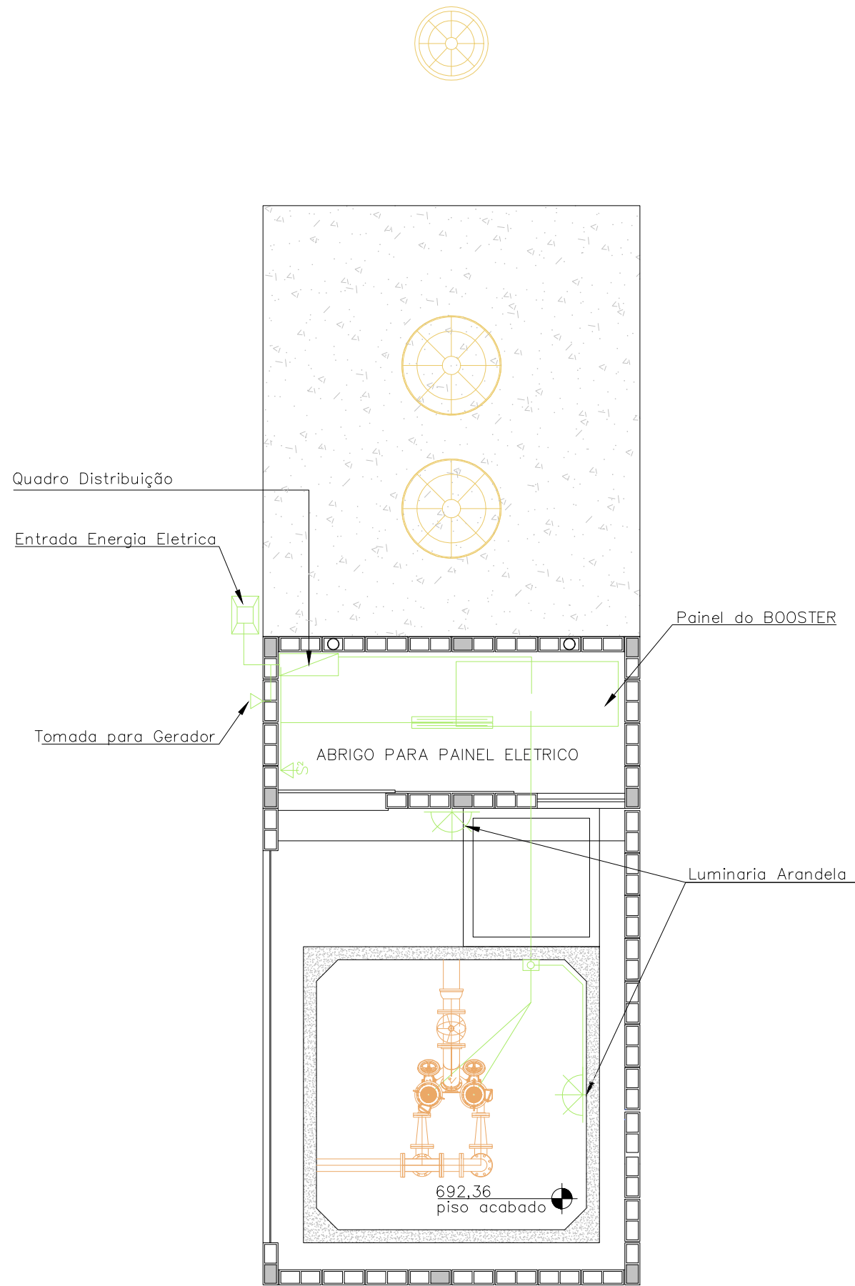
PLANTA BAIXA (ELETRICA) ESCALA_1/50
