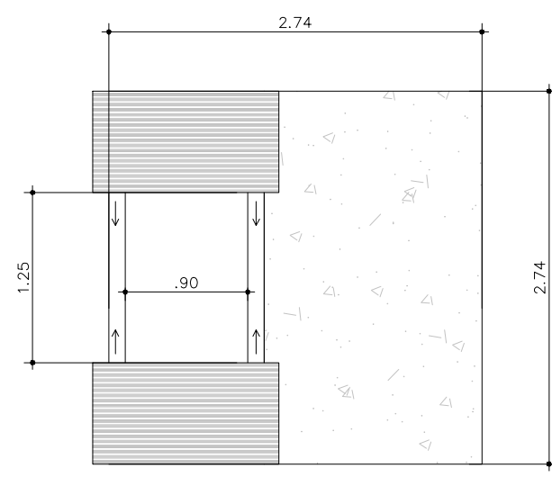
Det. Tampa Abrigo BOOSTER ESCALA_1/50
