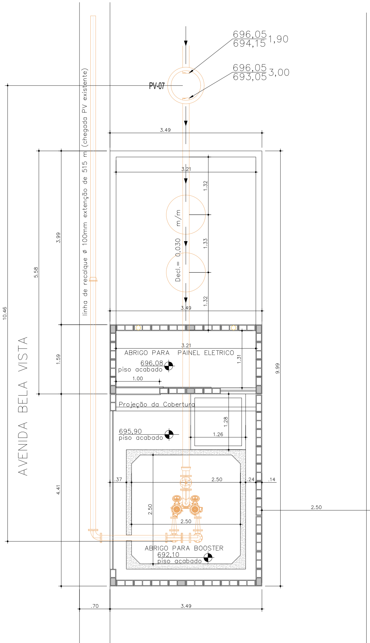
PLANTA BAIXA ESCALA_1/50
