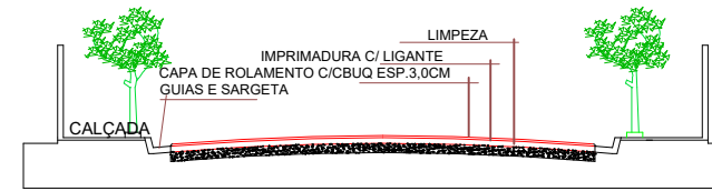
PROJETO BASICO- RECAPEAMENTO ASFALTICO COM CBUQ SEÇÃO TRANSVERSAL ( PERFIL ) S/ ESCALA
