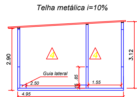
PISTA DE MALHA Corte CC Esc. 1:100
