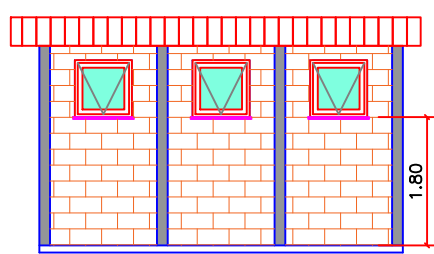
PISTA DE MALHA Fachada lateral - Vista C Esc. 1:100
