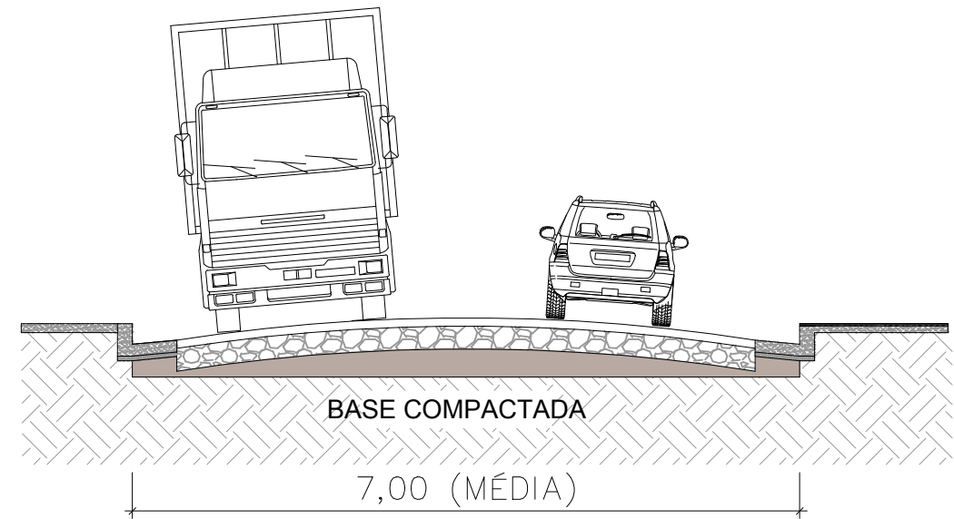
DETALHE - ARRUEAMENTO
