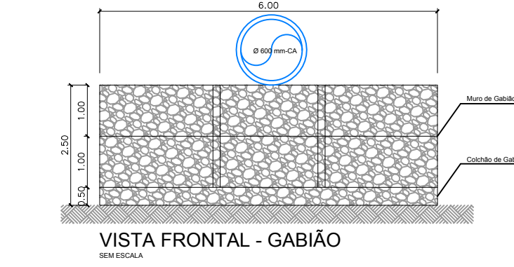
DETALHE 01 - GABIÃO
