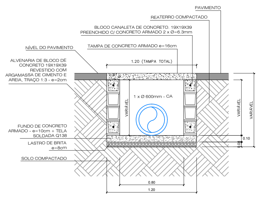
CORTE AA - DETALHE BOCA DE LOBO SIMPLES
