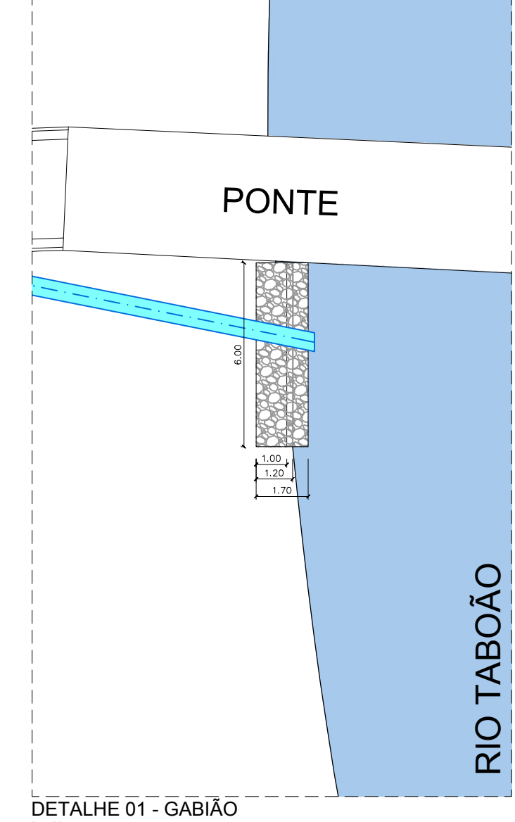
DETALHE 01 - GABIÃO
