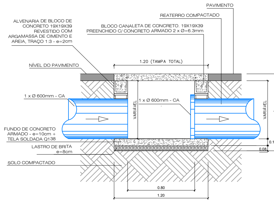
CORTE BB - DETALHE BOCA DE LOBO SIMPLES
