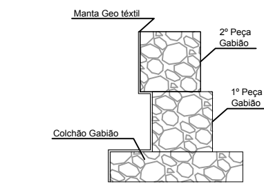
VISTA LATERAL - GABIÃO
