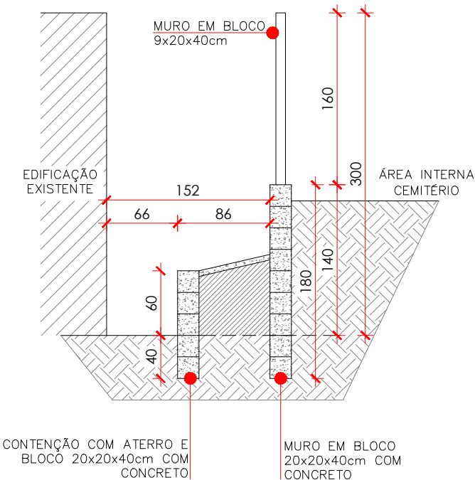
CORTE ESQUEMÁTICO MURO NOVO ESC.: 1/50
