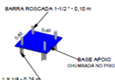
DETALHE - 02
