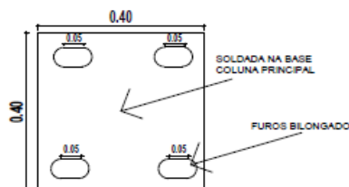
DETALHE - 01
