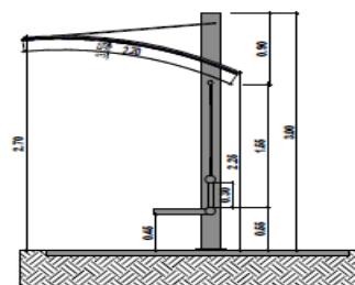
CORTE B
