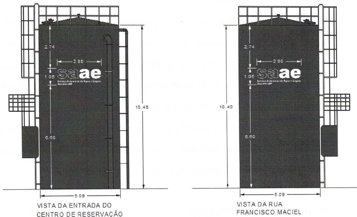
Imagem 01 – Vistas do reservatório
