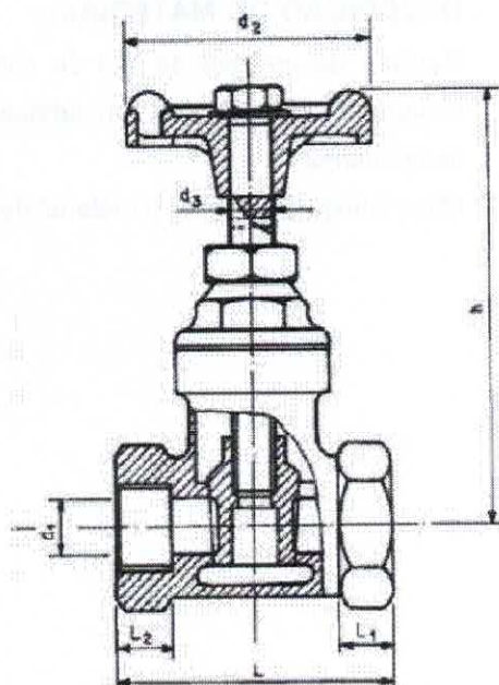
Dimensões do registro de gaveta
