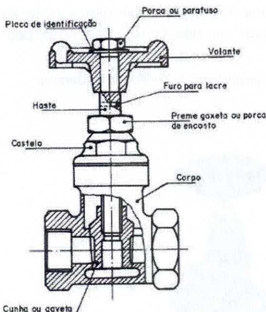
Descrição do registro de gaveta
