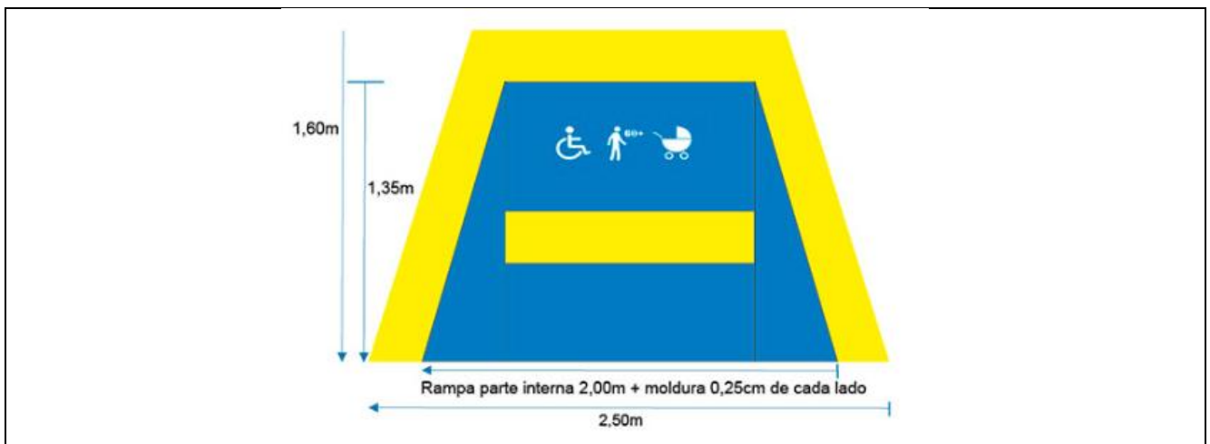
Detalhamento sinalização horizontal
