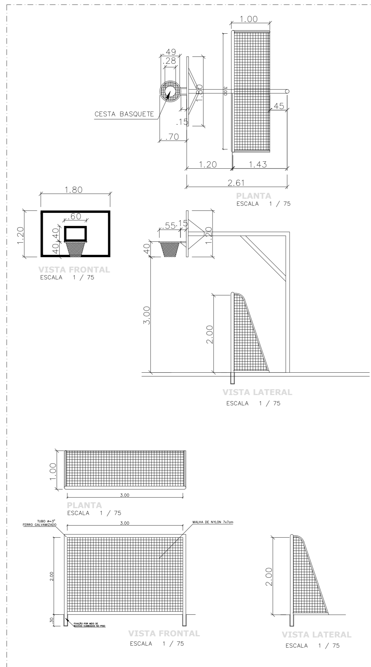
DETALHE – TRAVE E CESTA DE BASQUETE ESC. 1:100
