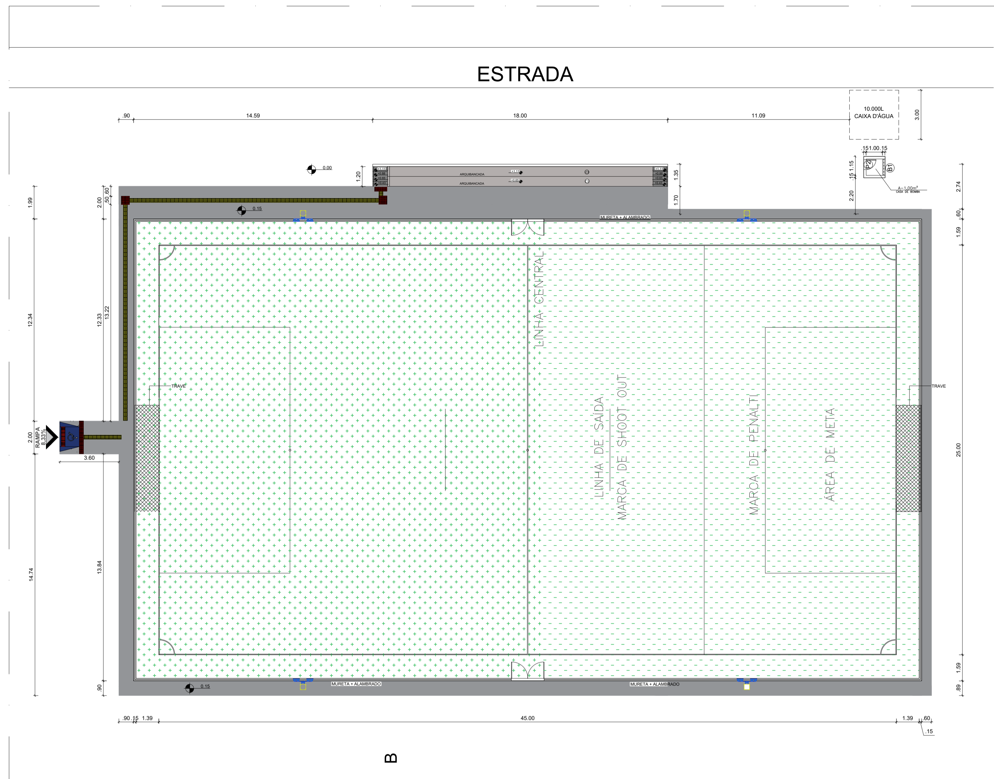
01 PLANTA BAIXA GERAL ESCALA: 1/100
