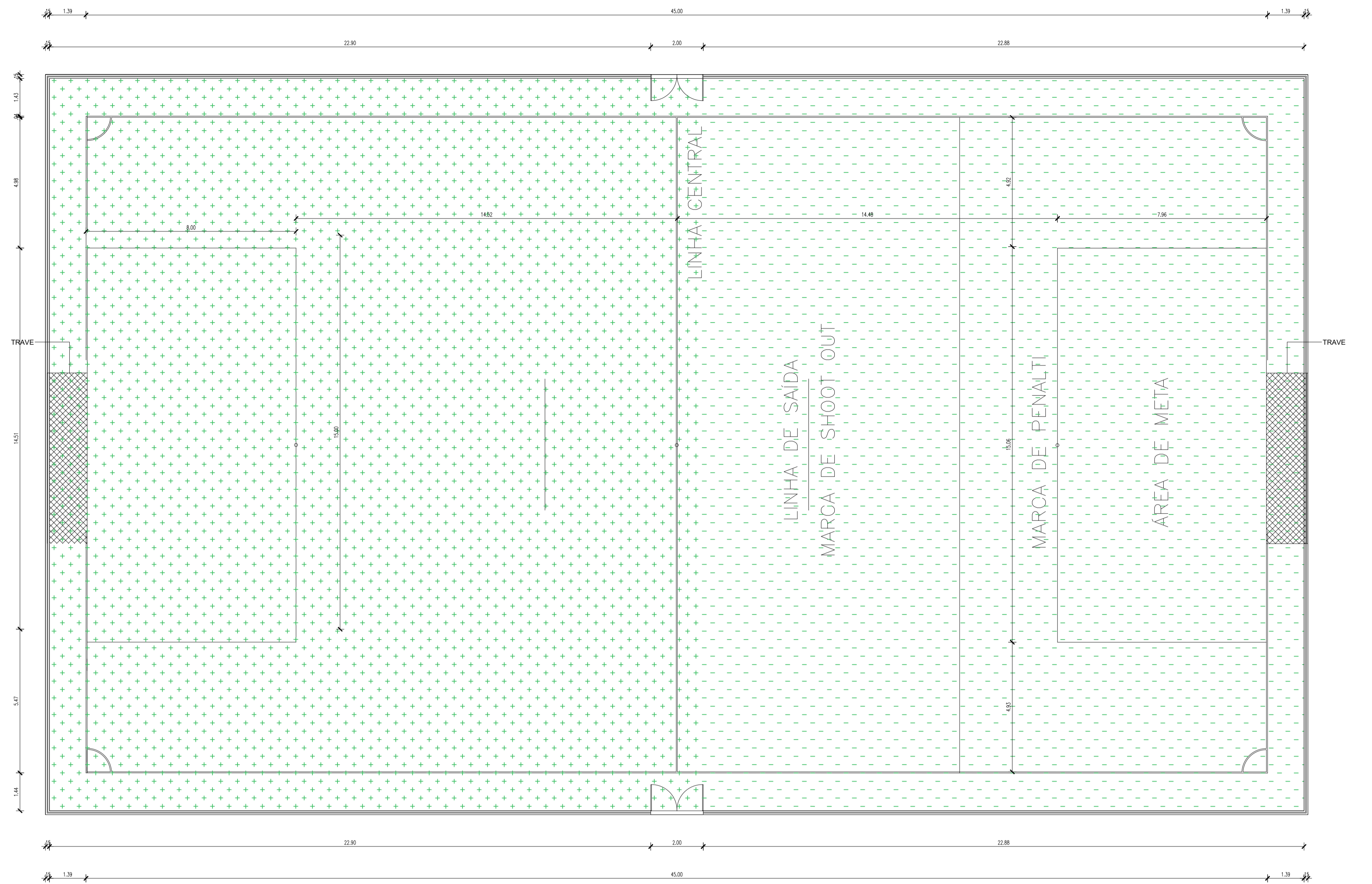
01 PLANTA BAIXA ESCALA: 1/75
