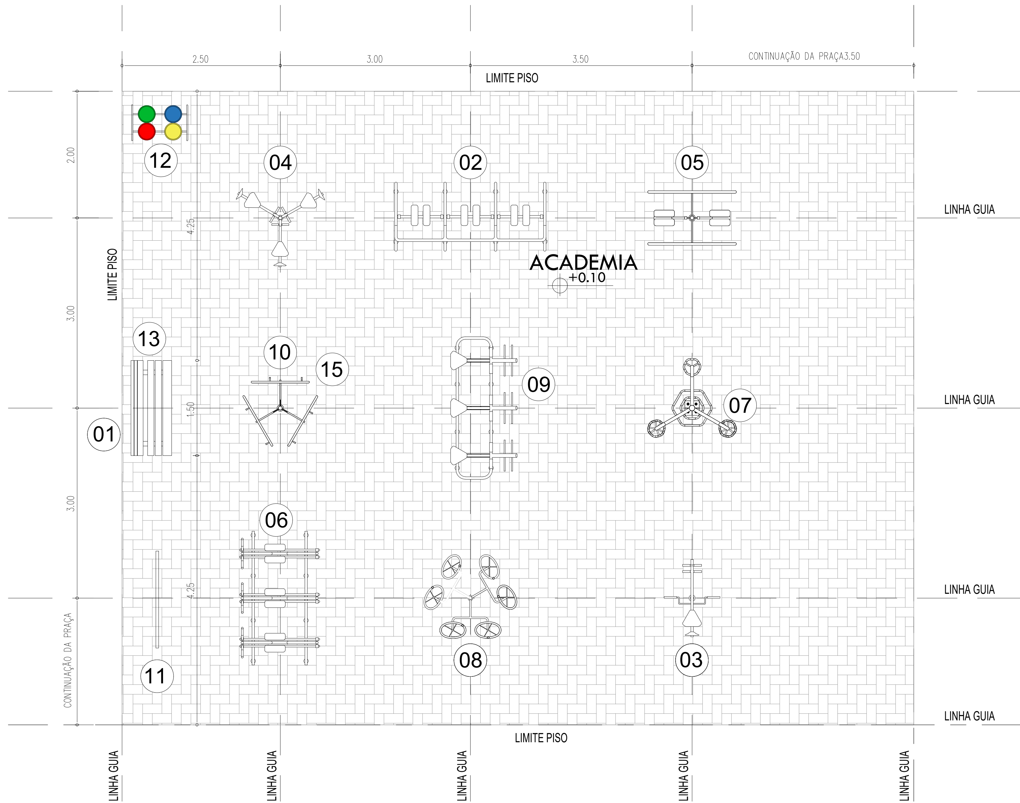
PLANTA BAIXA ACADEMIA ESCALA 1/50
