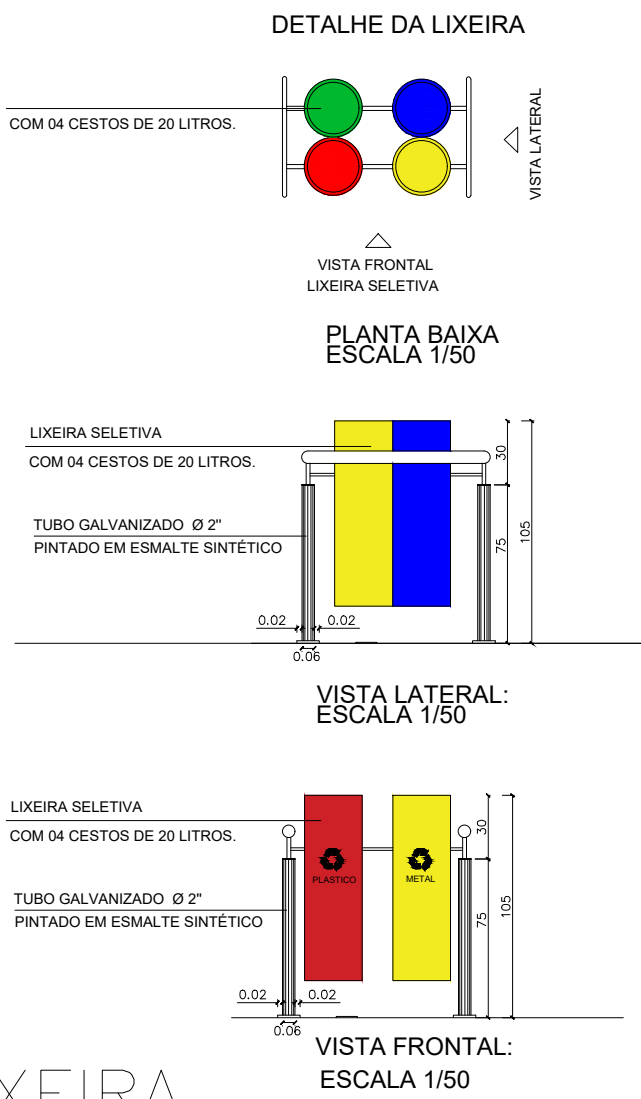
DETALHE LIXEIRA ESCALA 1/50
