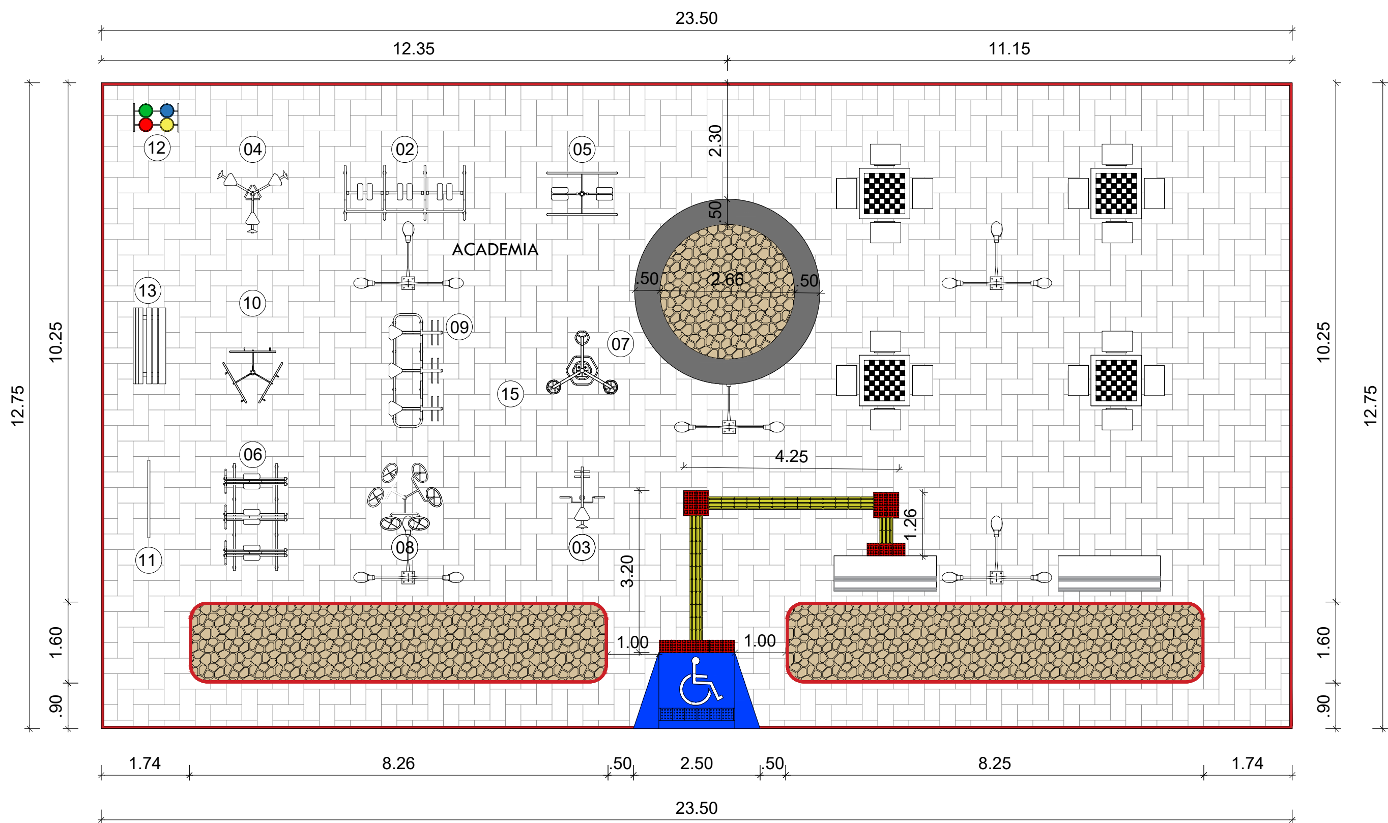
PLANTA BAIXA PRAÇA ESCALA 1/100
