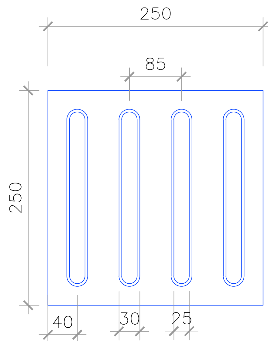
PISO TÁTIL DIRECIONAL (LARGURA DA FAIXA = 25 cm)
