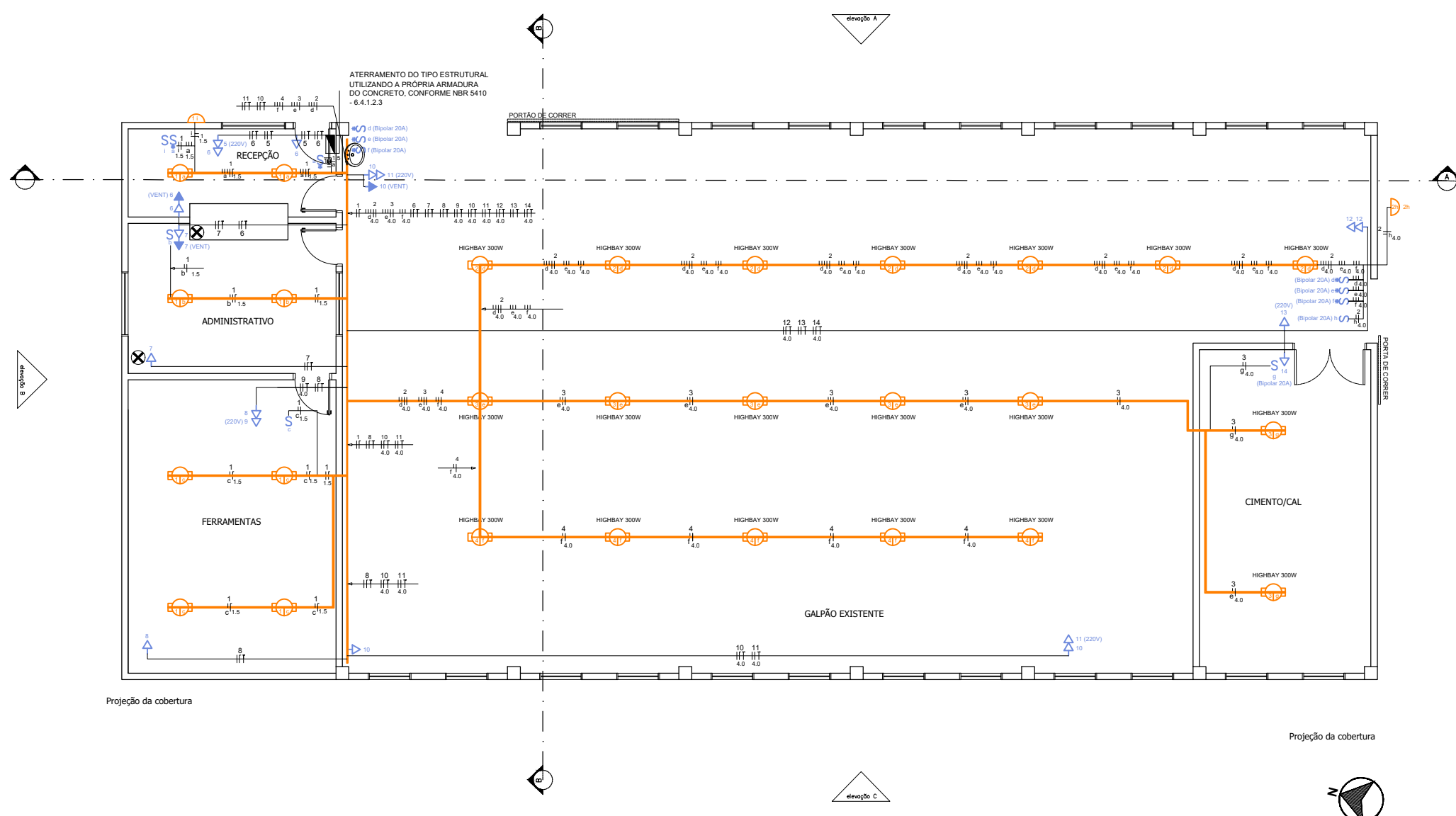
PROJETO BÁSICO ELÉTRICA - ALMOXARIFADO ESC. 1/125
