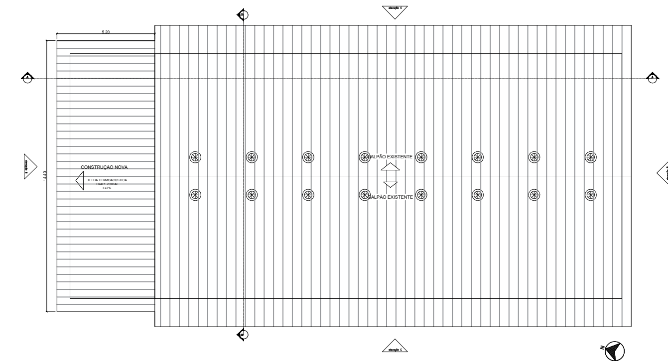
PLANTA COBERTURA - ALMOXARIFADO ESC. 1/200
