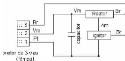
Figura 1 - Esquema de ligação elétrica do Kit Removível
