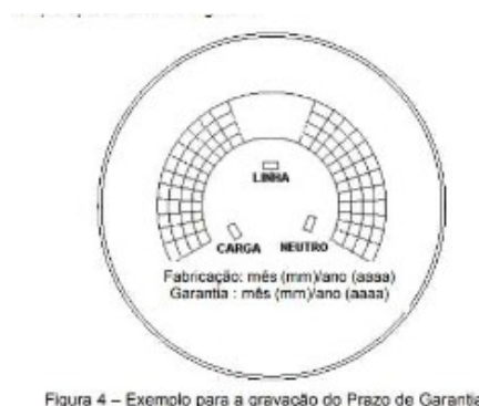
Figura 4 – Exemplo para a gravação do Prazo de Garantia
