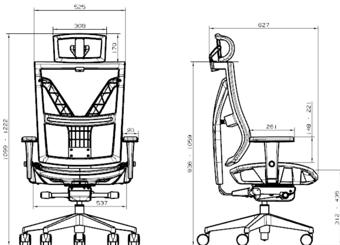
Figura 1 - Desenho técnico da poltrona ergonômica tipo presidente
