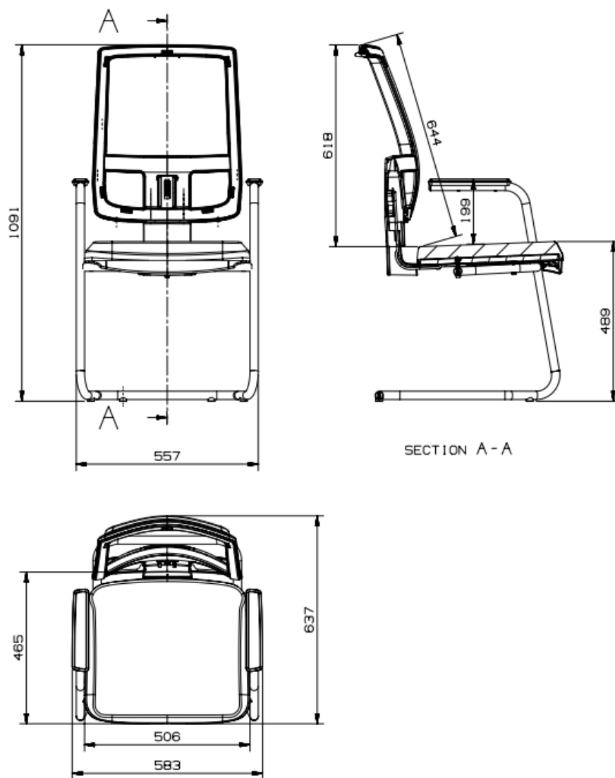
Figura 5 - Desenho técnico da poltrona tipo diretor
