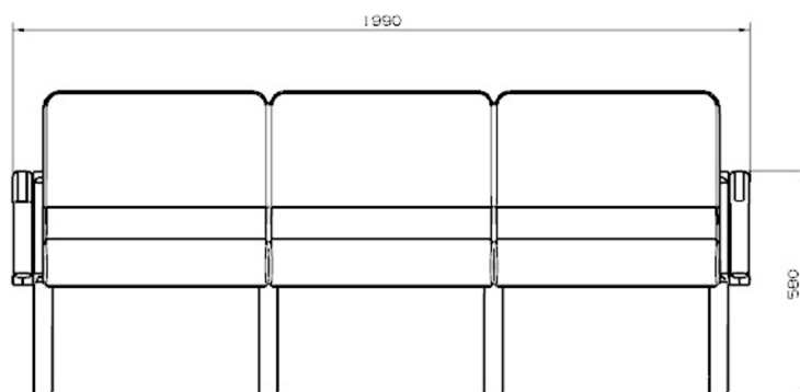
Figura 7 - Desenho técnico do sofá de 3 (três) lugares
