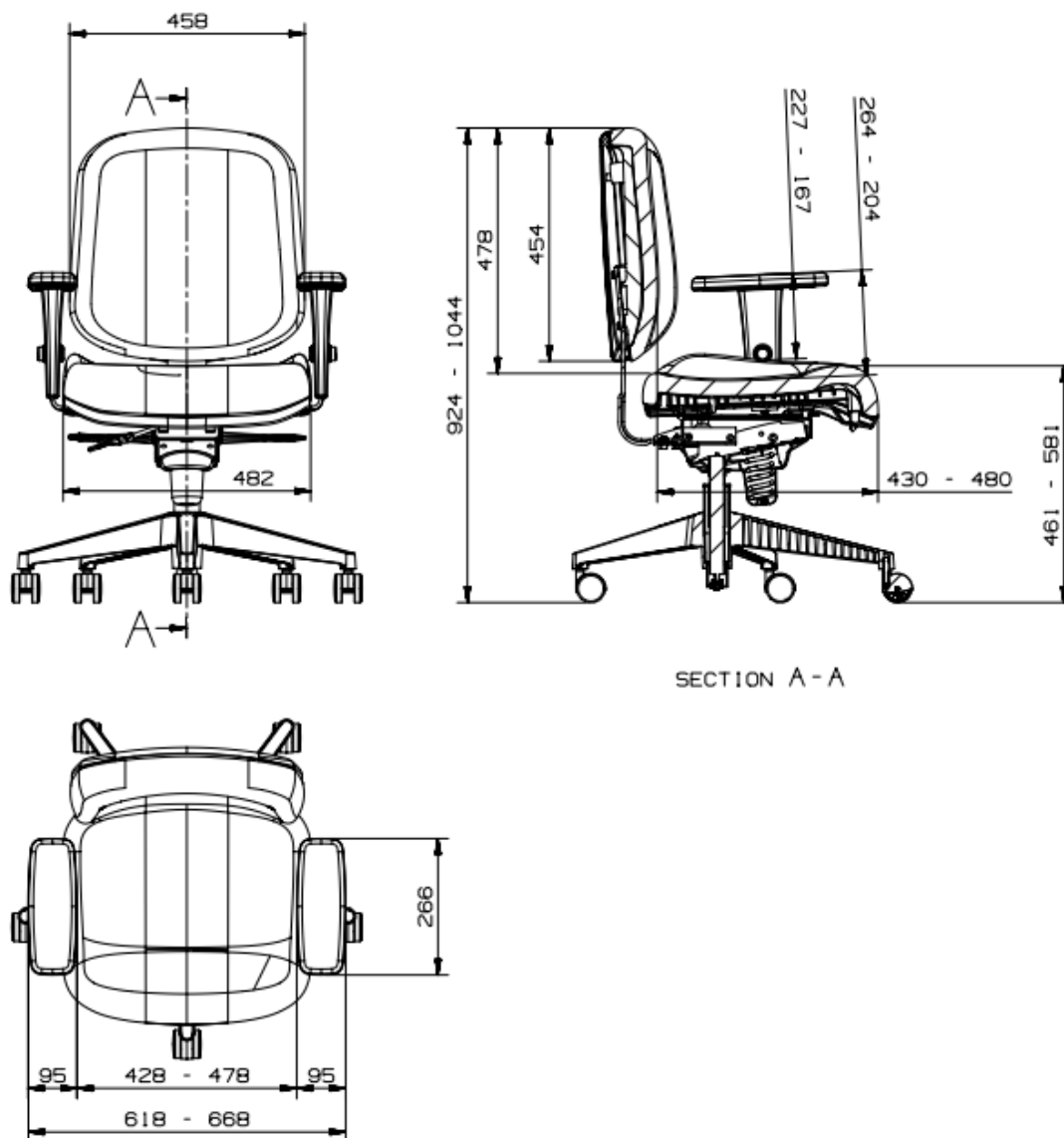
Figura 3 - Desenho técnico da poltrona ergonômica tipo diretor
