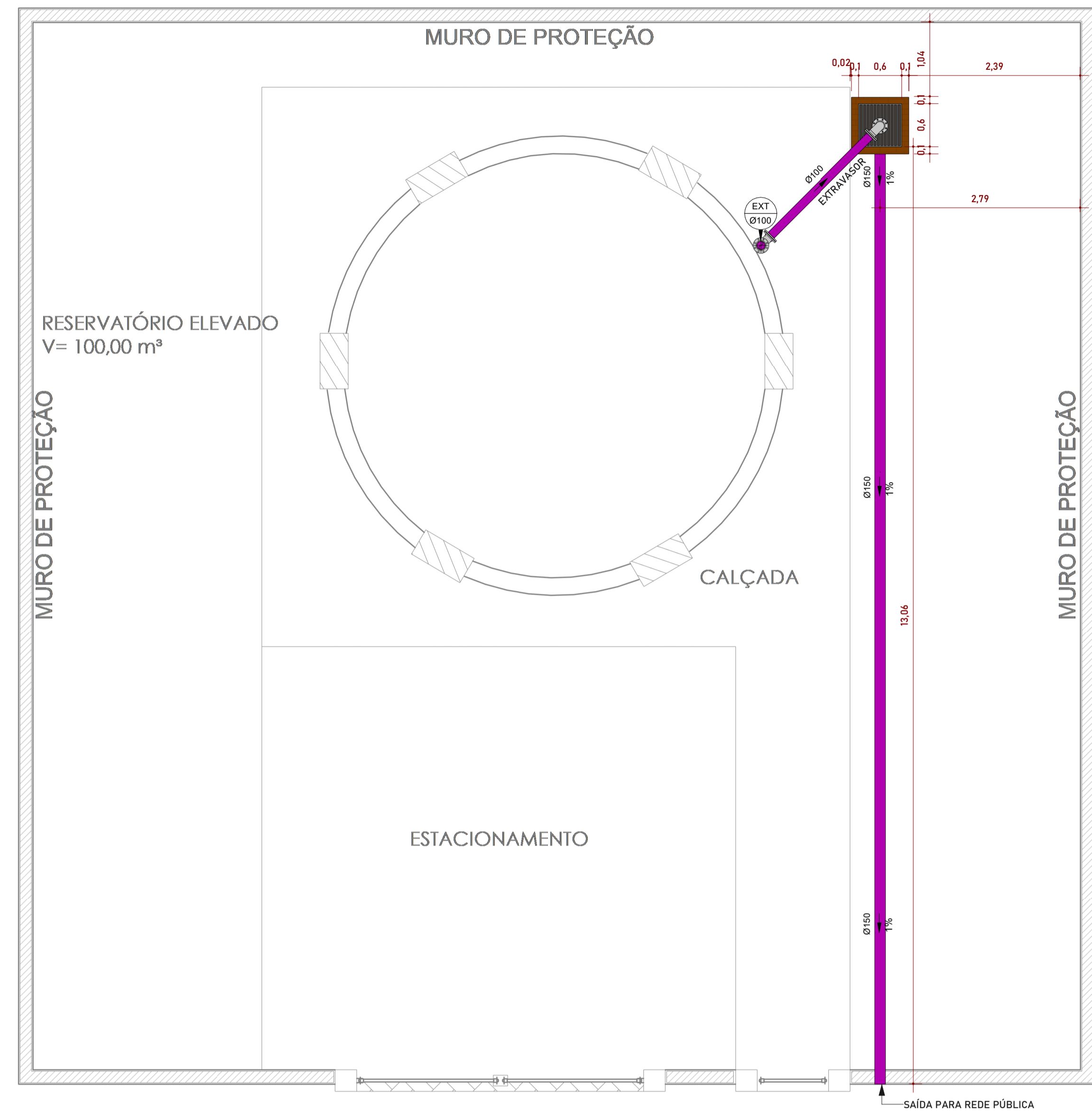
1 PAV. TÉRREO (PLV) Escala: 1:50
