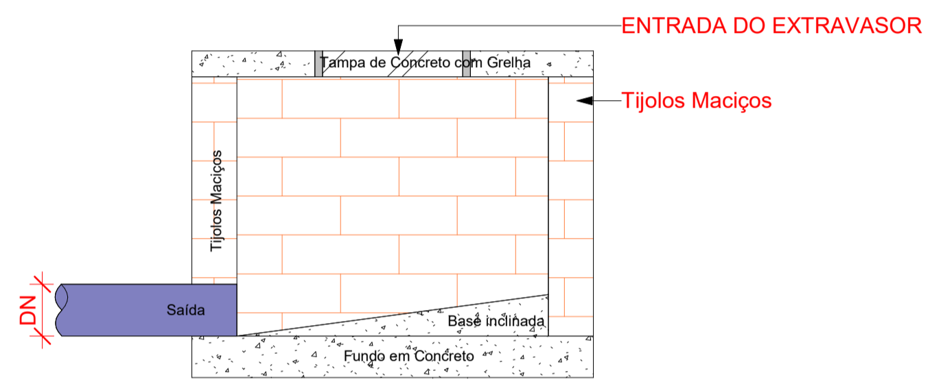
Corte lateral - Caixa de Passagem Pluvial 1 : 10
