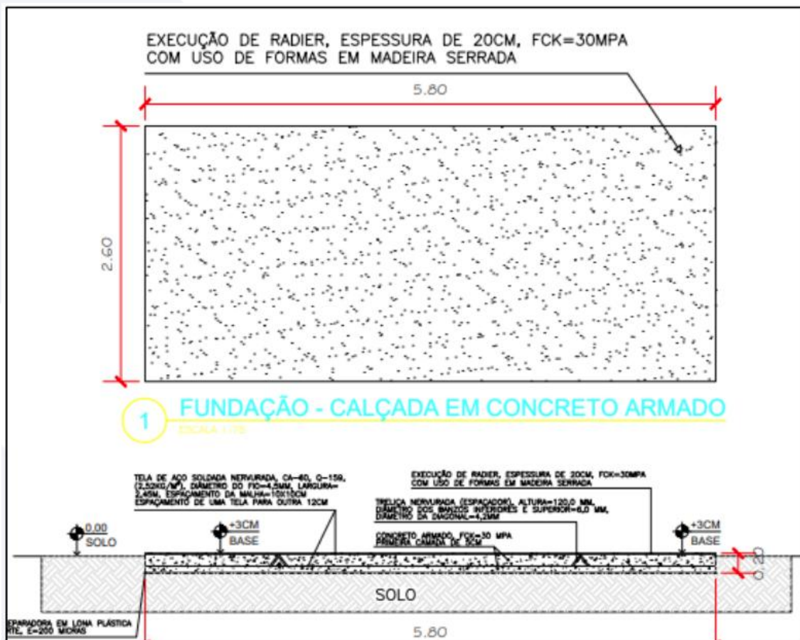
Imagem 7: Elemento de Fundação - Radier
