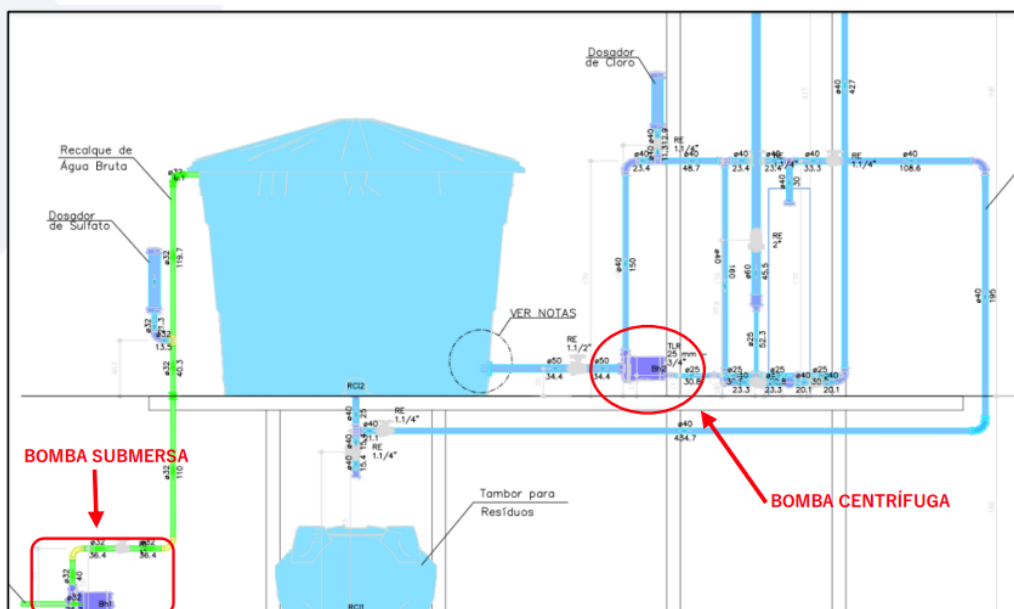
Imagem 6: Instalações Eletromecânicas
