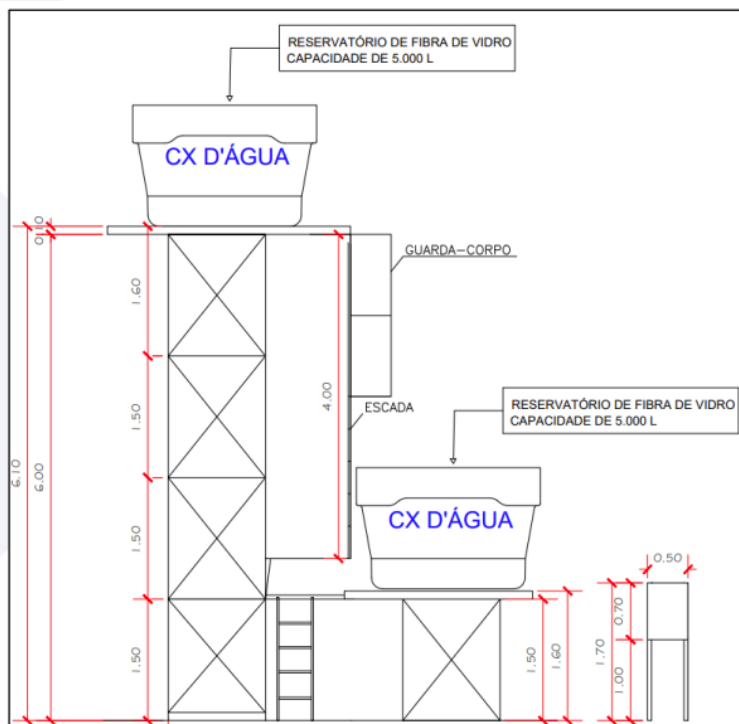
Imagem 8: Estrutura Metálica do Sistema Água Boa
