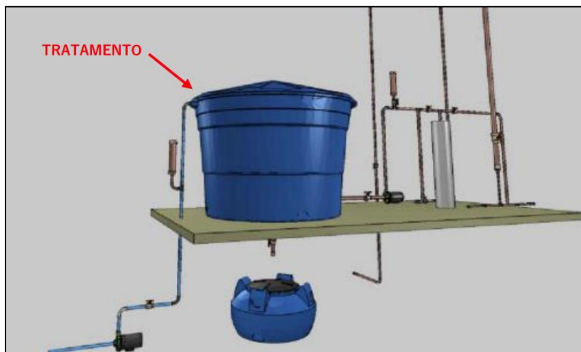
Imagem 4: Reservatório Inferior – Tratamento
