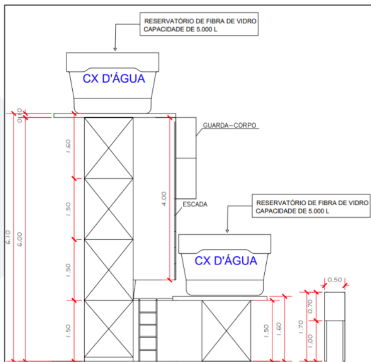
Imagem 9: Estrutura Metálica do Sistema Água Boa
