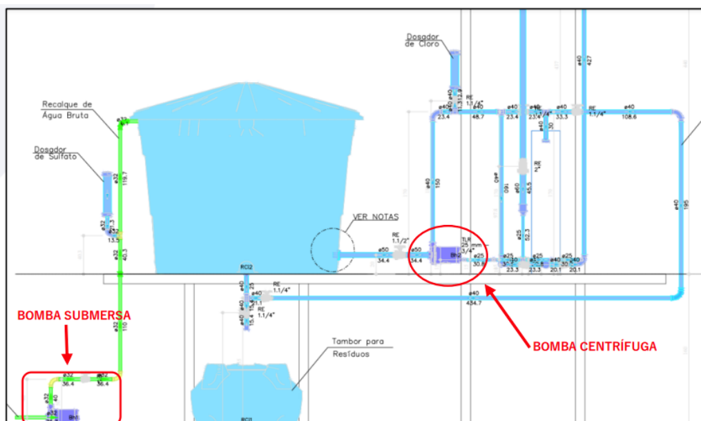
Imagem 7: Instalações Eletromecânicas
