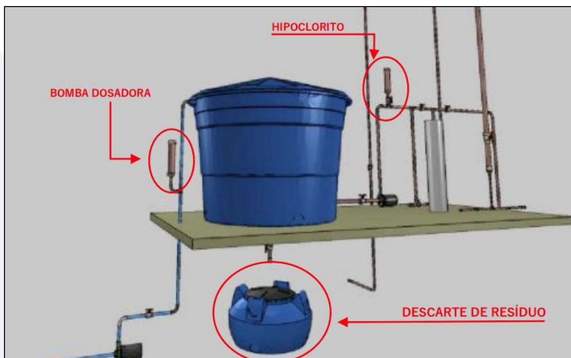
Imagem 6: Componentes do Sistema Água Boa
