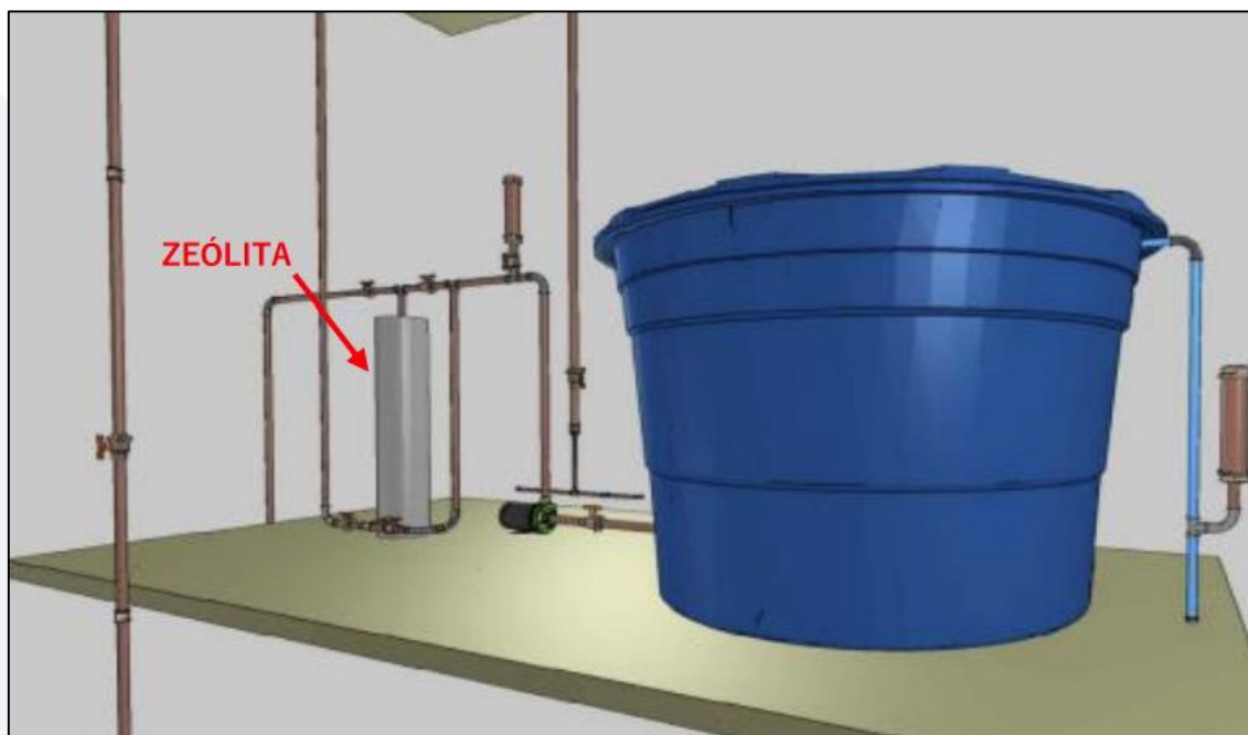
Imagem 5: Elemento Filtrante Clinoptilolita - Zeólita
