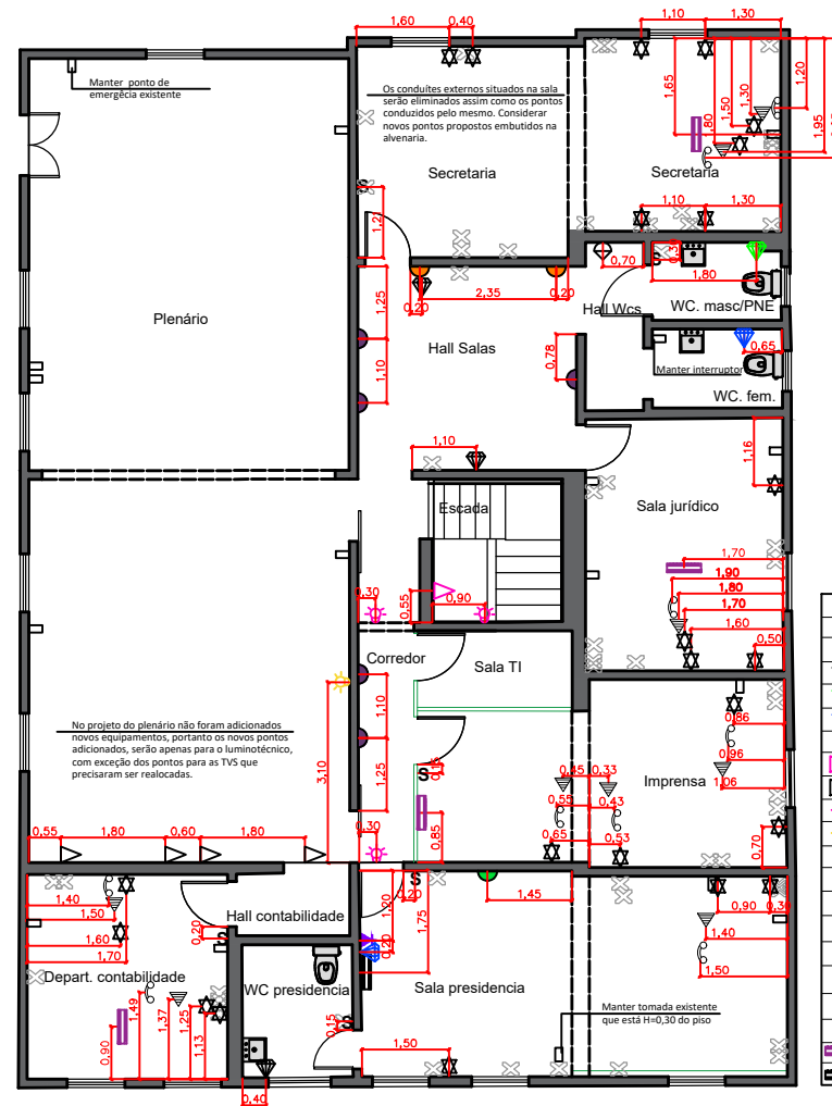
Planta baixa pontos elétricos Escala 1/100
