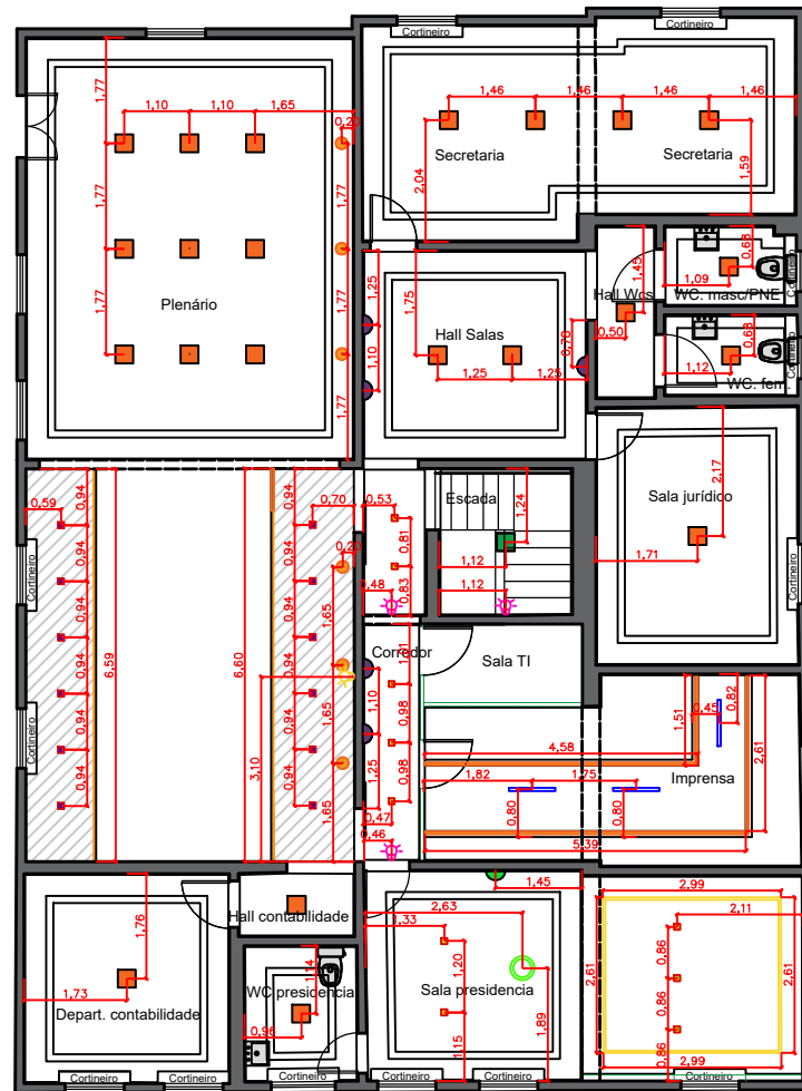
Planta baixa pontos de iluminação Escala 1/100
