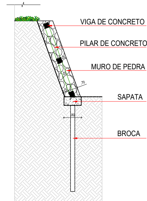
DETALHE _ MURO DE PEDRA S/ESCALA
