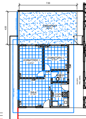
CASA DO CASEIRO À CONSTRUIR ESC.: 1:125
