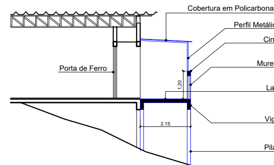
CORTE A ESC 1:75
