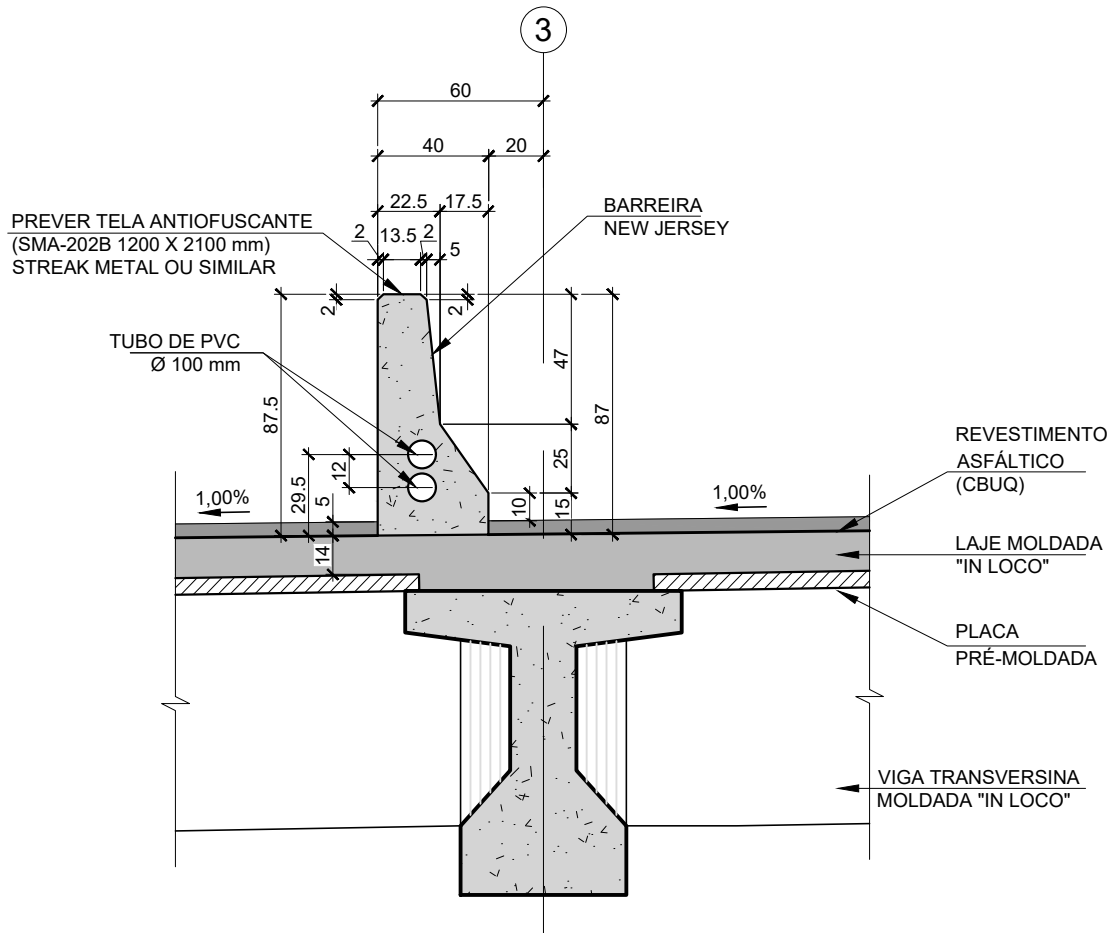
DETALHE DA BARREIRA NEW JERSEY / PINGADEIRA ESC.1:25
