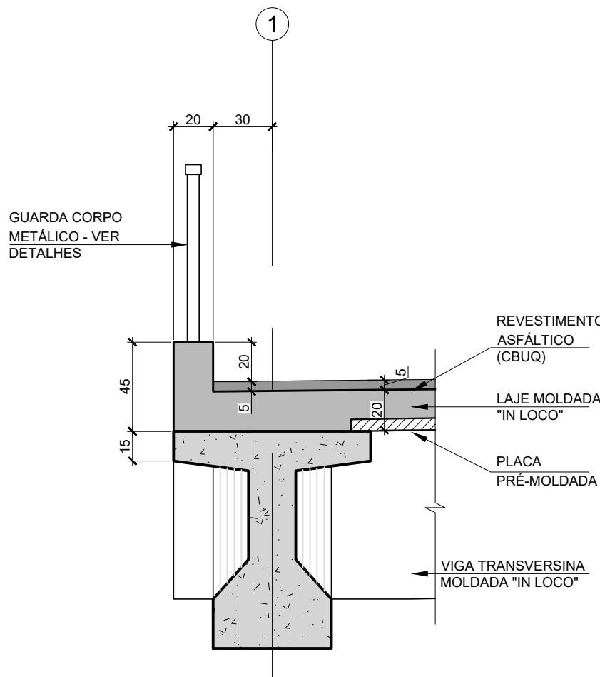
DETALHE DO GUARDA CORPO ESC.1:25
