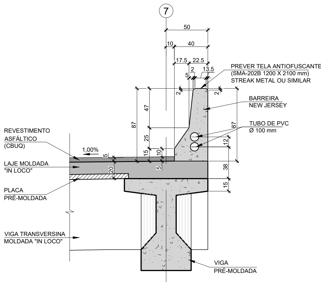
DETALHE DA BARREIRA NEW JERSEY / PINGADEIRA ESC.1:25
