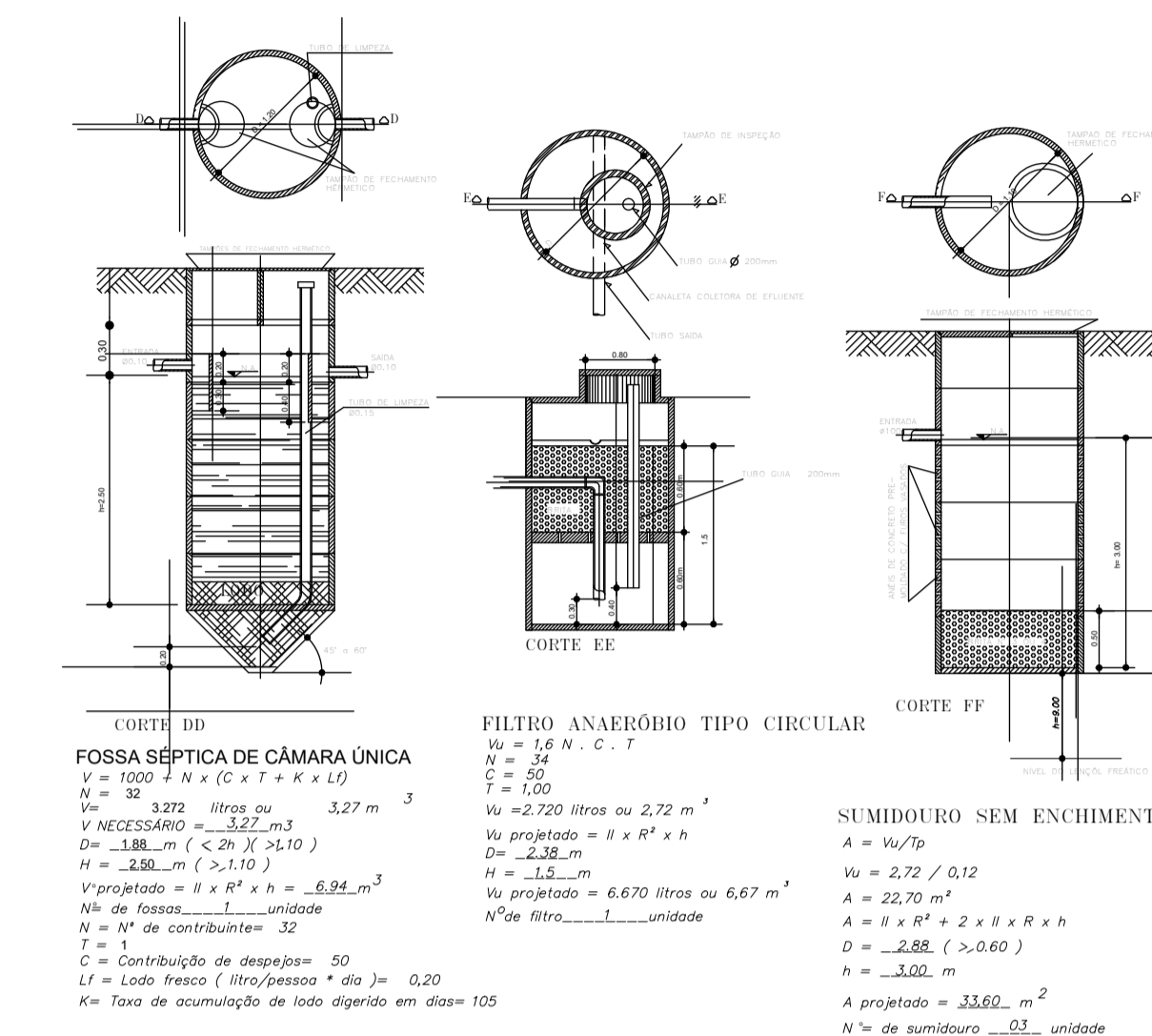
MEMORIAL DE CALCULO DE TANQUE SÉPTICO E EFLUENTES LÍQUIDOS conforme (NBR 7229/93 E NBR 13.969/97).
