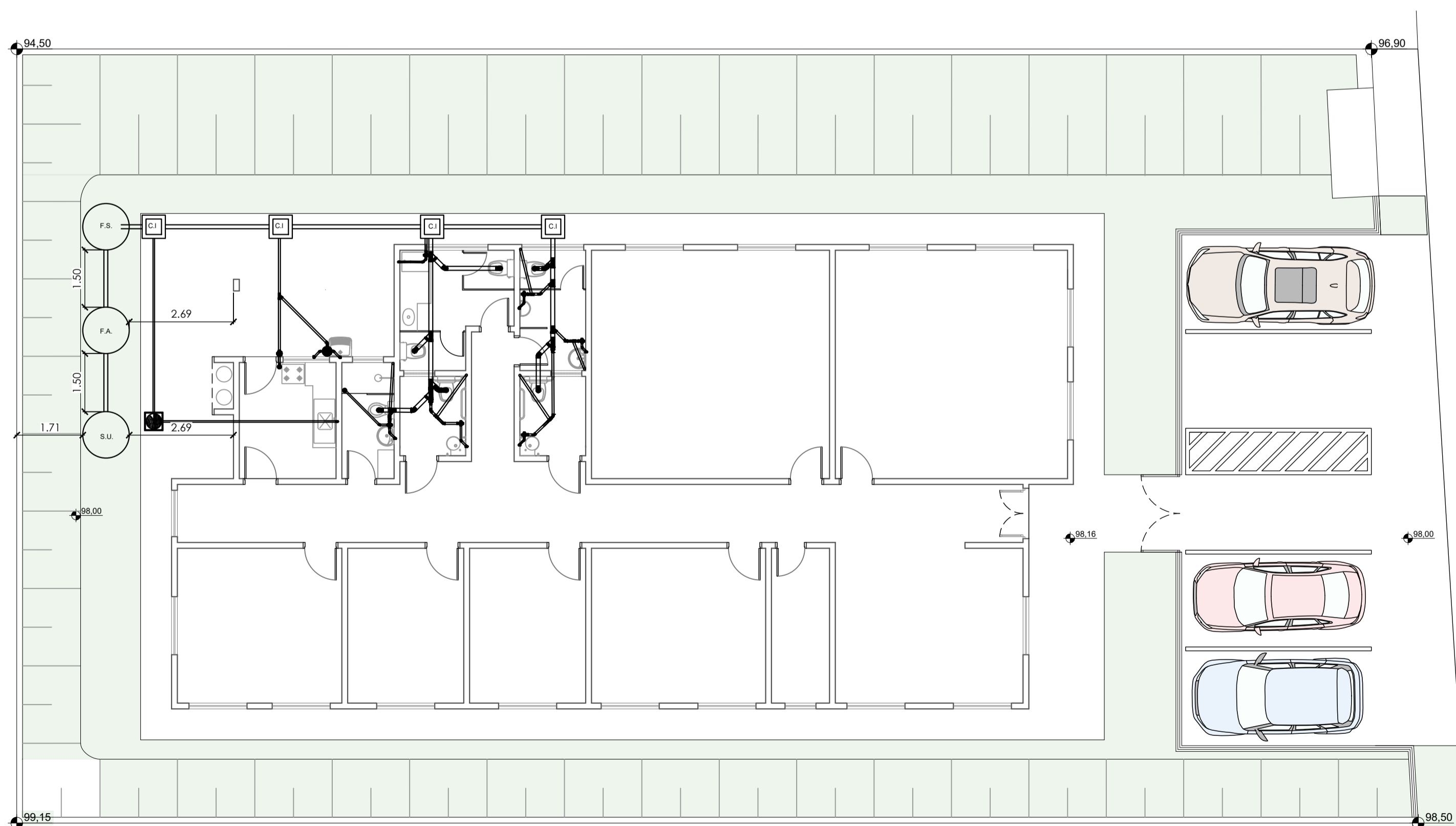
PLANTA PAV. TÉRREO | ESGOTO
