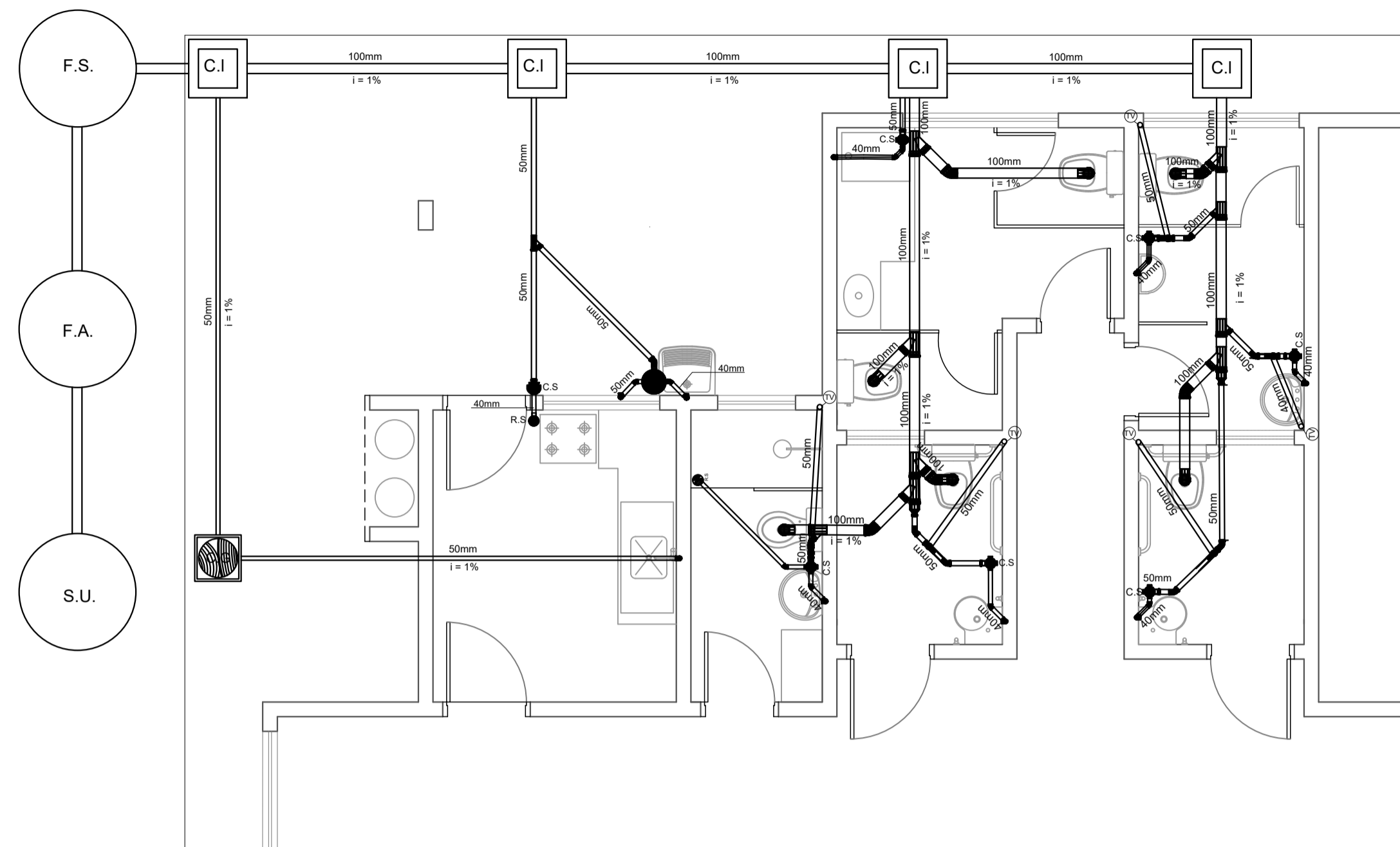
PLANTA DE ESGOTO
