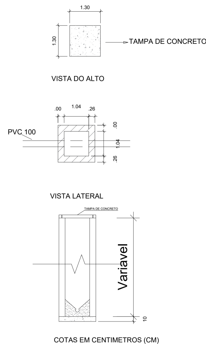
DETALHE DA CAIXA DE INSPEÇÃO - CI
