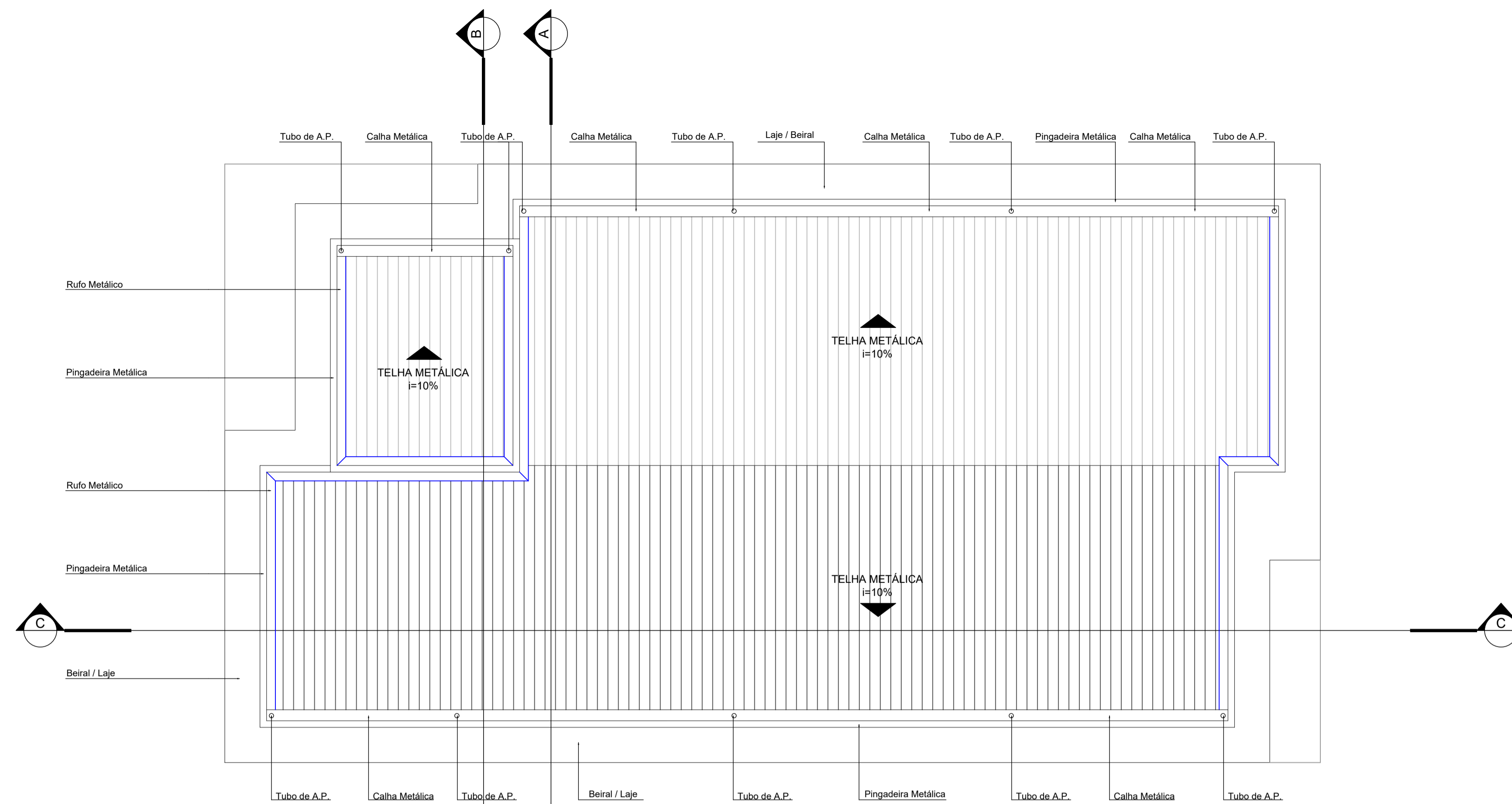
PLANTA DE COBERTURA ESC 1:75
